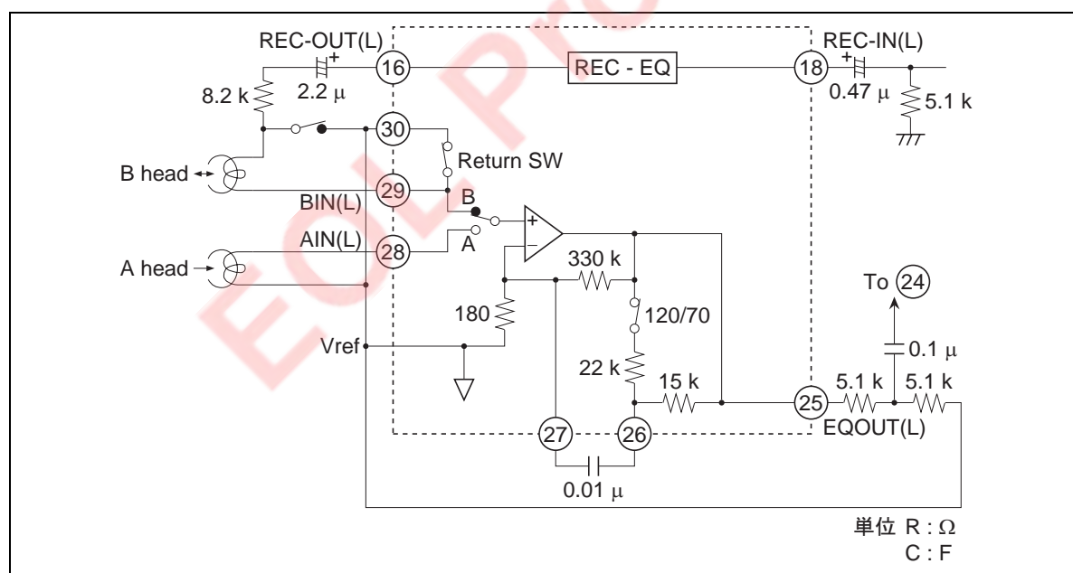
図 2 ブロックダイアグラム (Lch)
