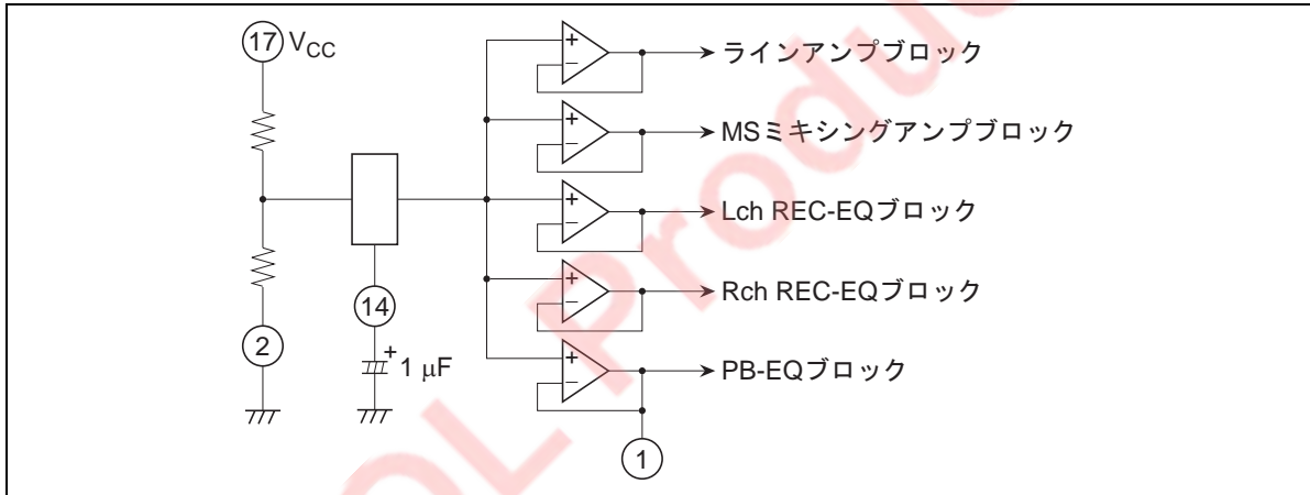
図 1 基準電圧回路
