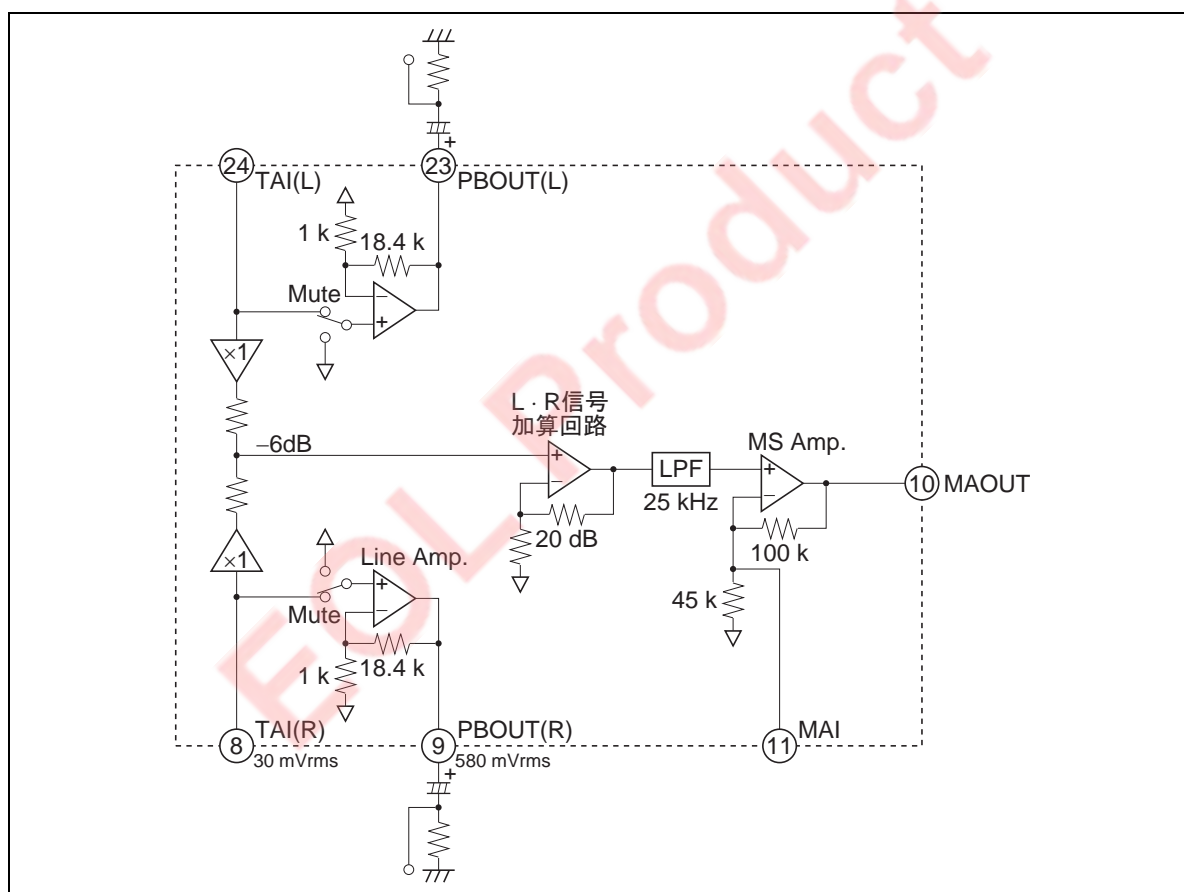
図4 ミュージックセンサミキシングアンプブロック
