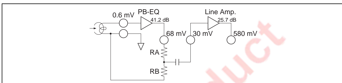
図 3 PB 系レベルダイアグラム (120 \mu s, 1kHz)
