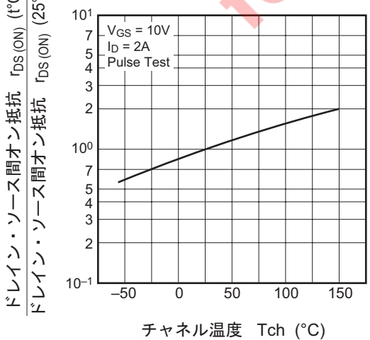
ドレイン・ソース間オン抵抗— チャンネル温度特性 (代表例)
