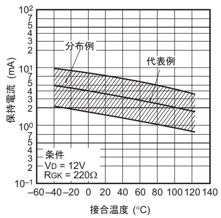
保持電流 - 接合温度
