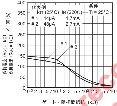
保持電流 - ゲート・陰極間抵抗
