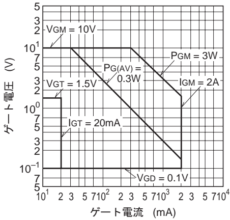
ゲート特性 (I, IIおよびIII)
