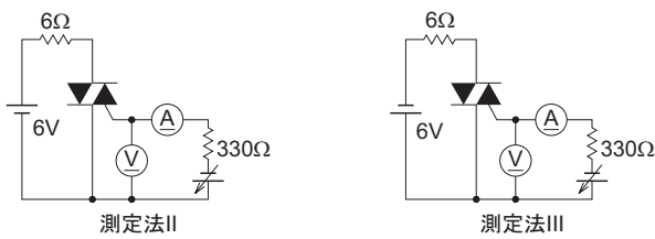
ゲートトリガ特性測定回路
