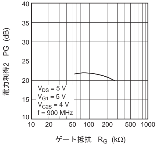
電力利得2対ゲート抵抗特性
