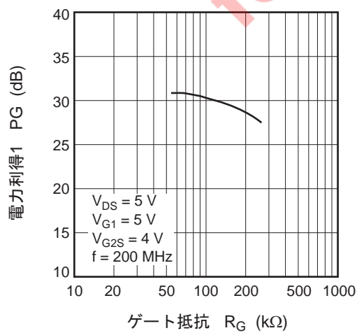
電力利得1対ゲート抵抗特性
