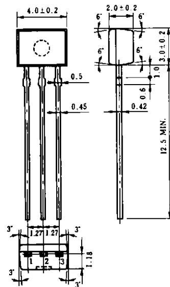
外形図 (単位: mm)
