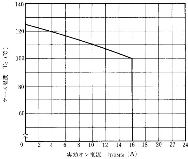
図11 T_c-I_{T(RMS)} 定格
