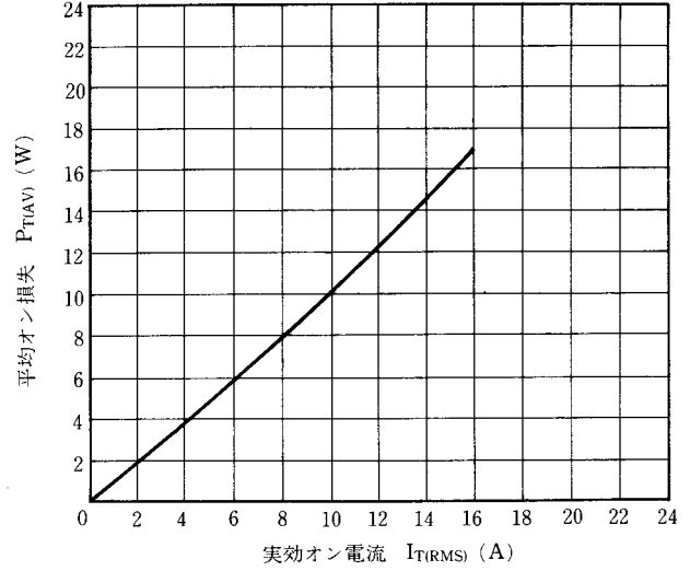
図10 P_{T(AV)}-I_{T(RMS)} 特性
