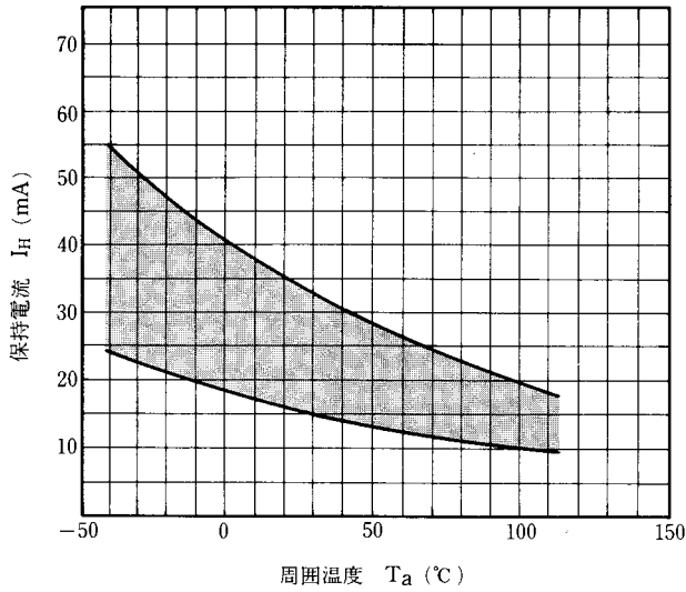
図9 I_H-T_a 特性例
