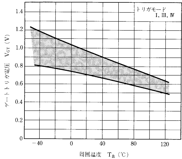
図6 V_{GT} - T_a 特性
