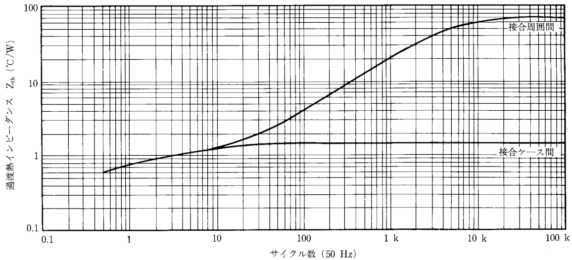
図13 Z_{th} 特性
