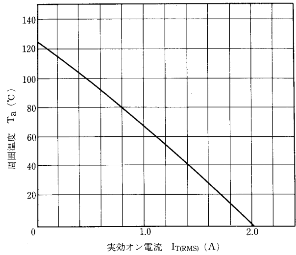
図12 T_a-I_{T(RMS)} 定格
