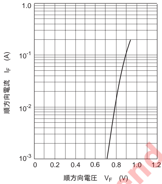
图1. 顺方向特性
