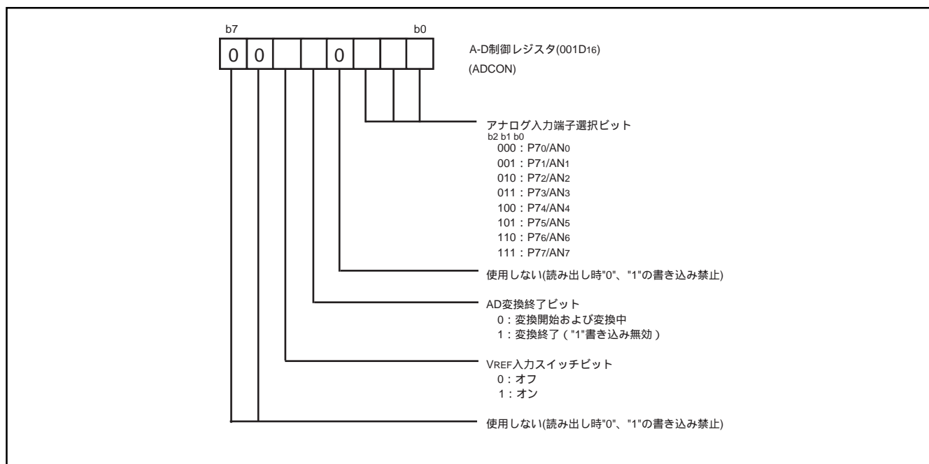
図48. A-D制御レジスタ
