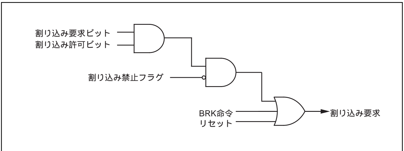
図19. 割り込み制御図
