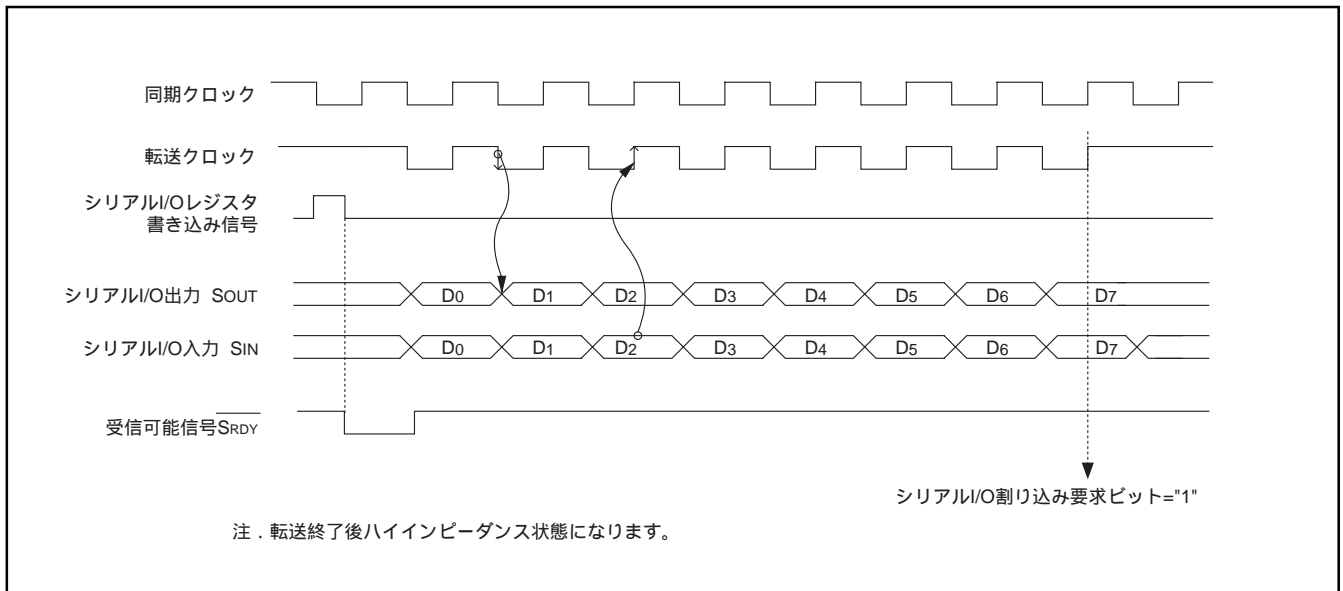
図28. シリアル/O動作タイミング図
