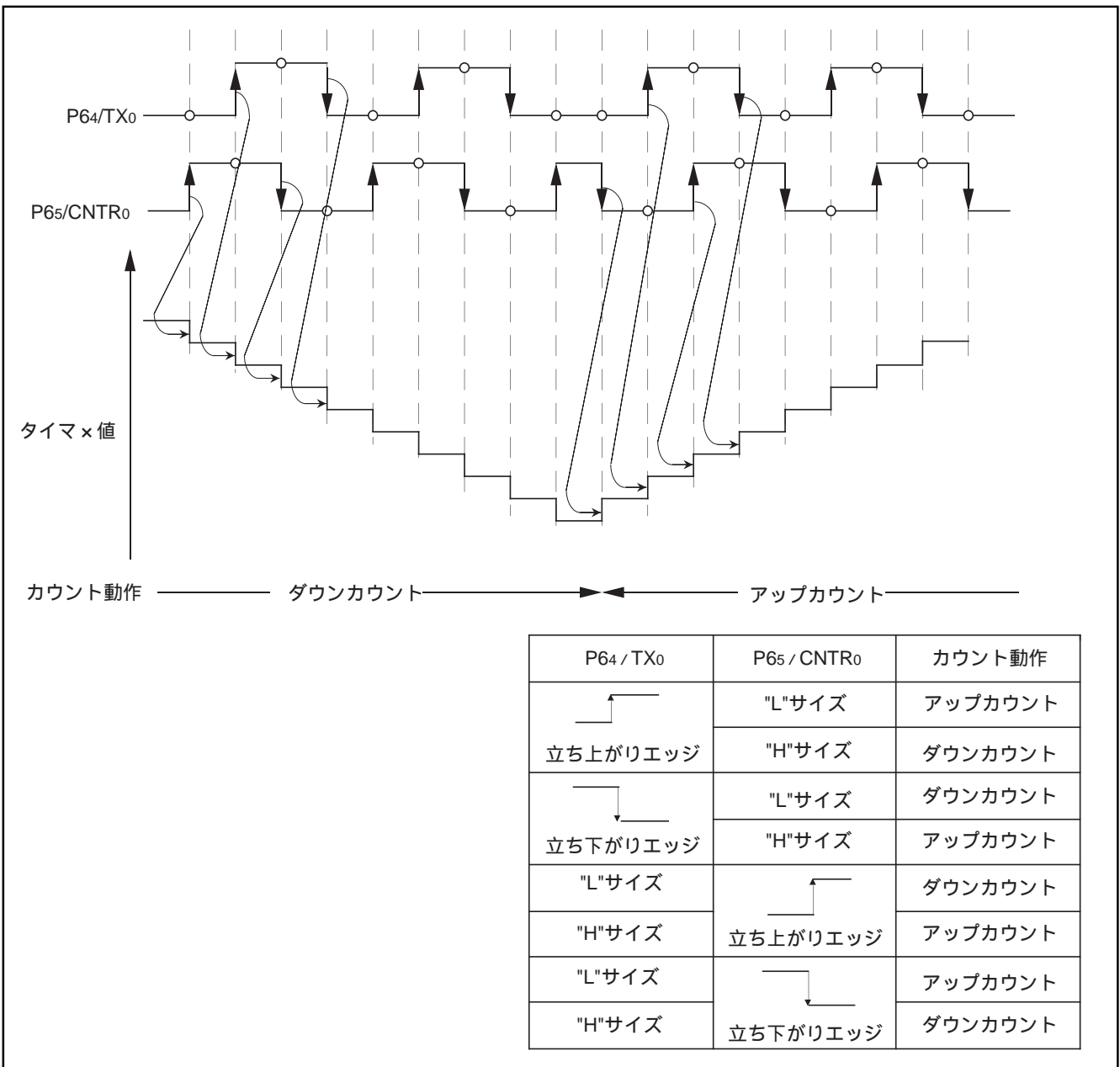
図23. タイマX二相パルス処理モード時のタイミングチャート
