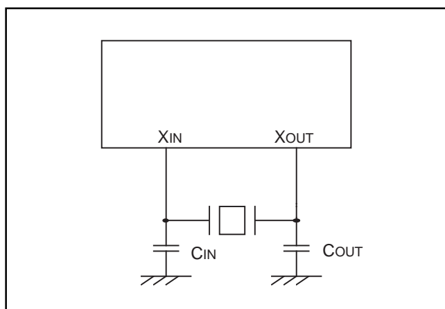
図54. 発振回路
