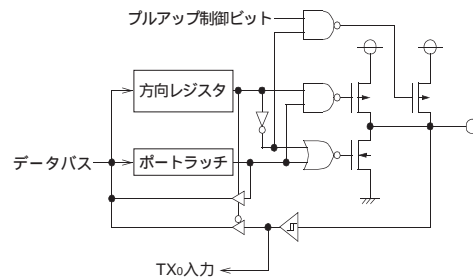
(12) ポート P64/TX0
