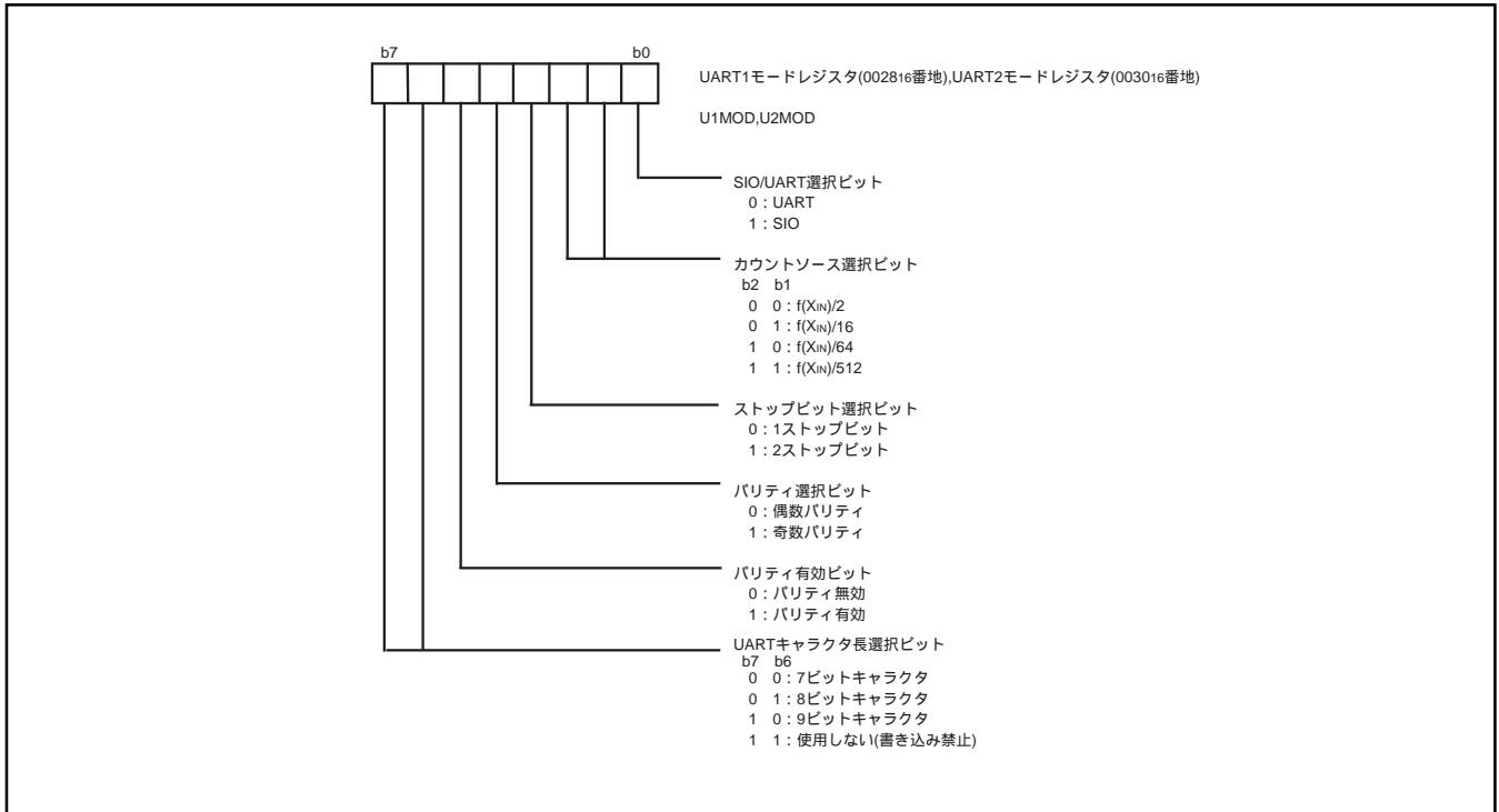
図31. UARTモードレジスタ
