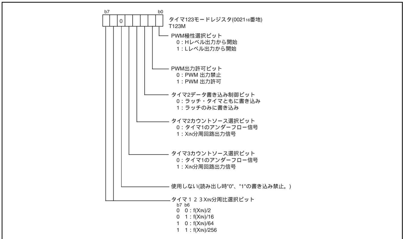
図26. タイマ123モードレジスタ
