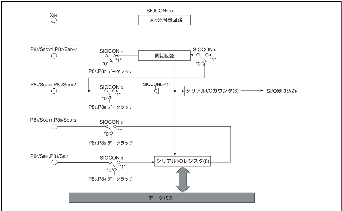
図27. シリアルI/Oブロック図
