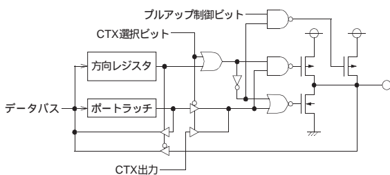
(15) ポート P41/CTX
