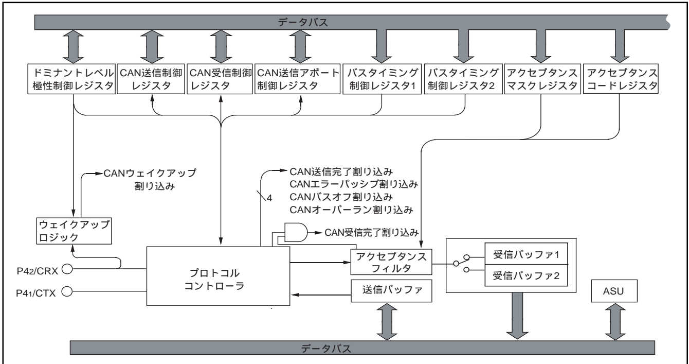
図34. CANコントローラブロック図
