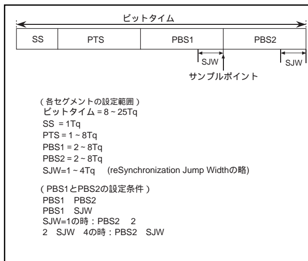
図38. ビットタイミング
