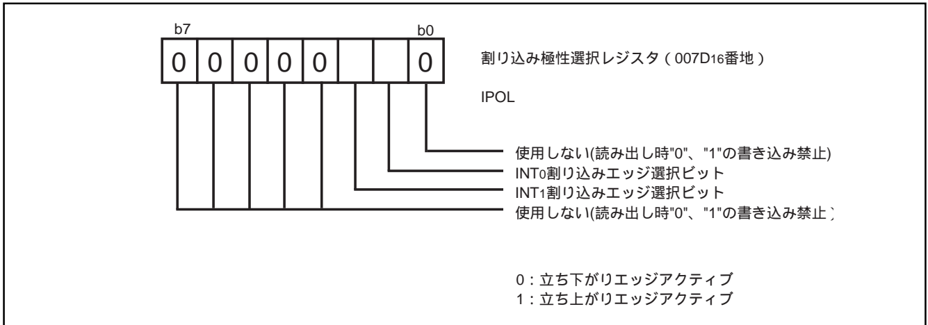
図18. 割り込み極性選択レジスタ
