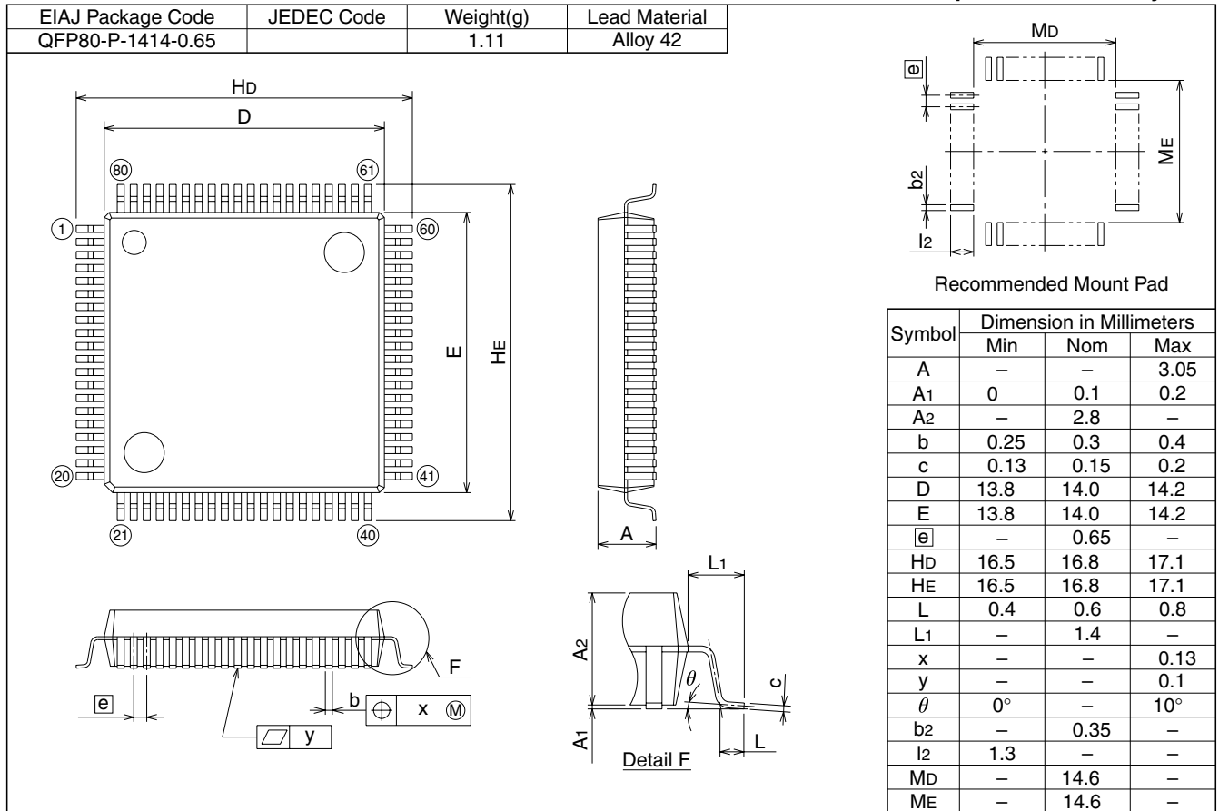
図60. パッケージ外形寸法図(80P6S-A)
