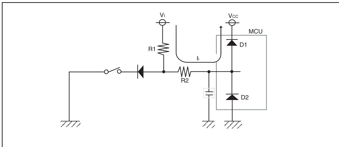
図56. レベルシフト入力回路構成図
