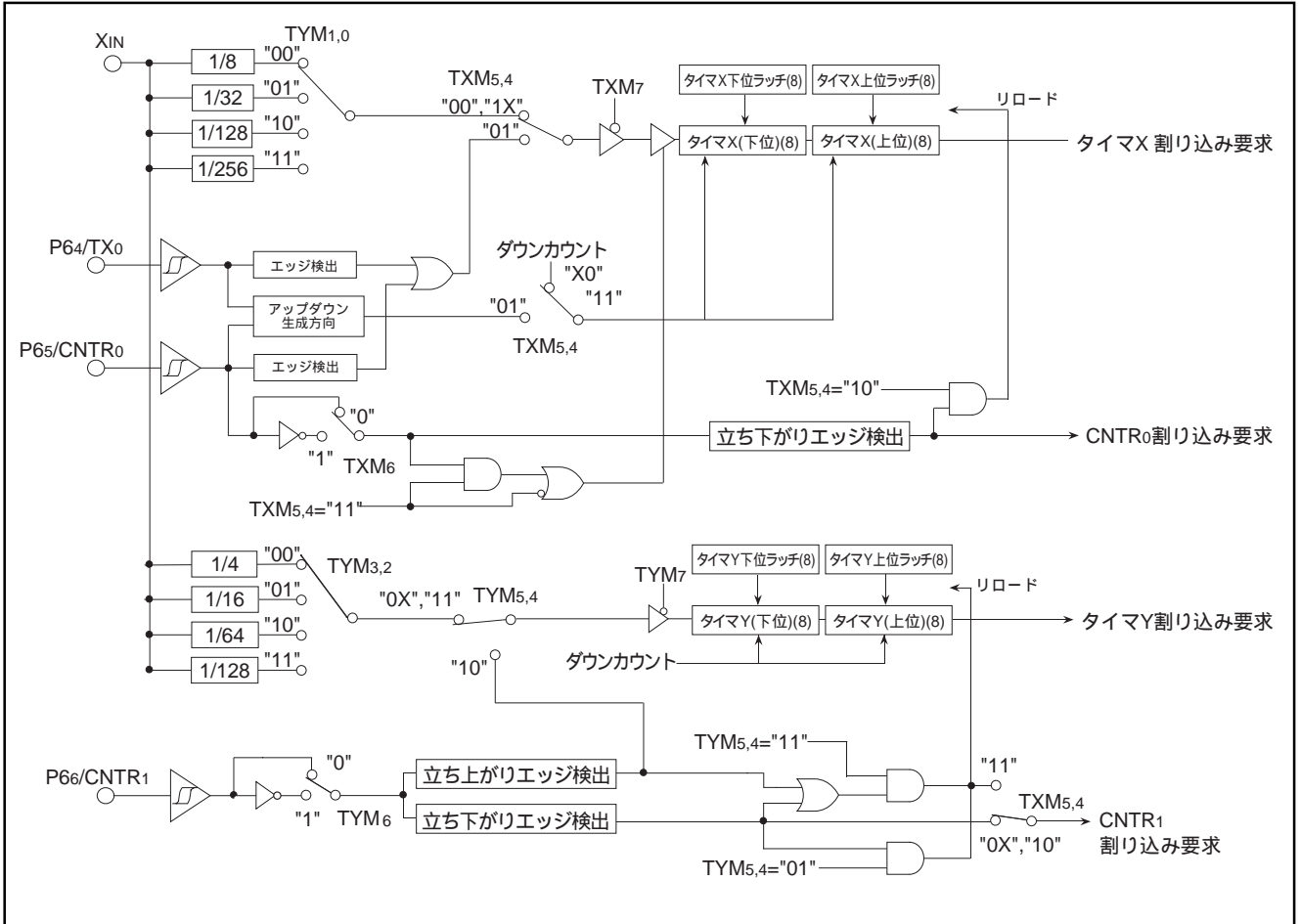
図21. タイマX,タイマYブロック図
