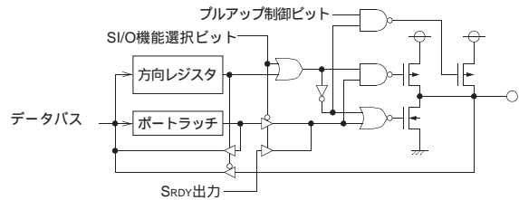
(12) ポート P64/TX0
