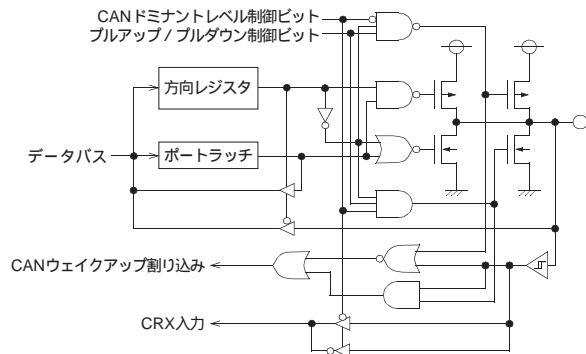
(16) ポート P42/CRX
