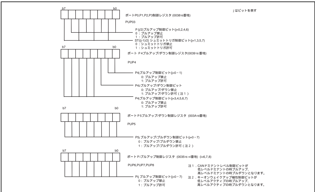
図15. ポートプルアップ / プルダウン制御レジスタ
