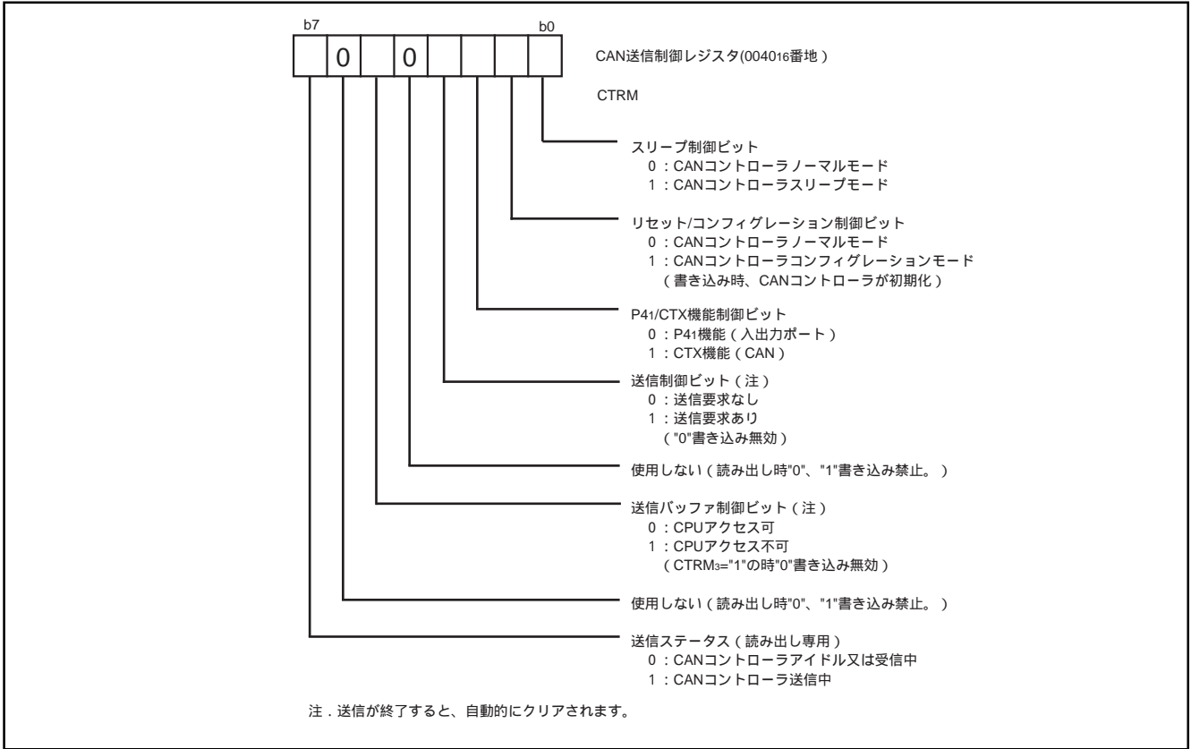
図39. CAN送信制御レジスタ
