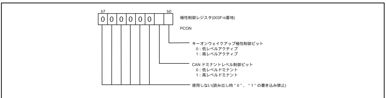
図16. 極性制御レジスタ
