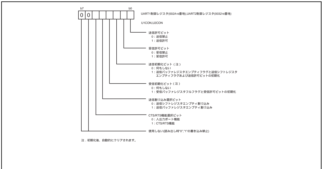
図32. UART制御レジスタ
