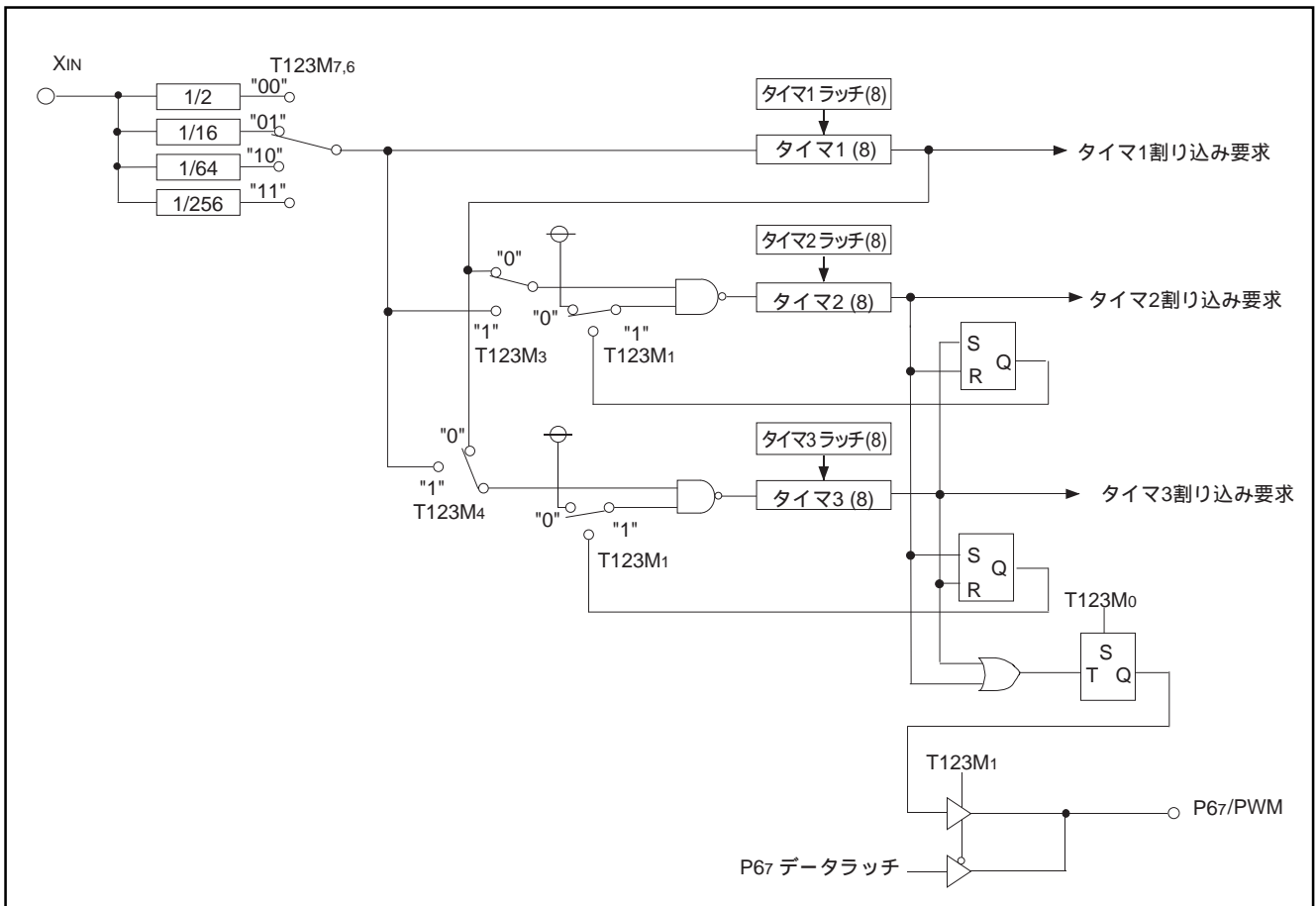
図25. タイマ123ブロック図
