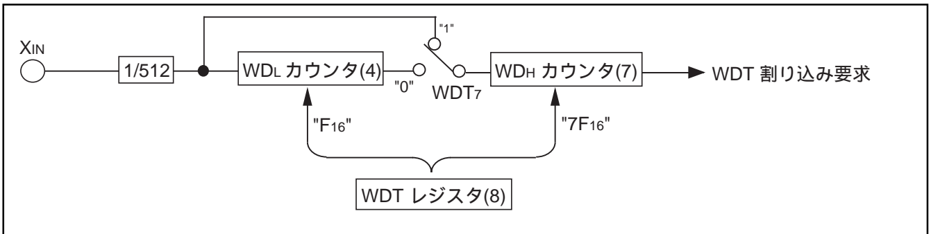
図49. ウォッチドッグタイマブロック図
