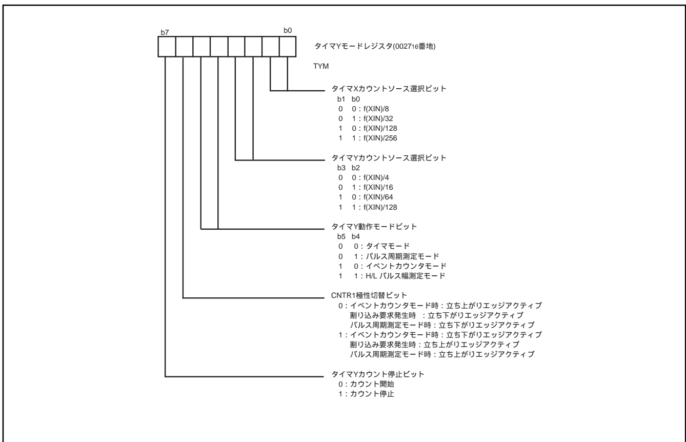
図24. タイマYモードレジスタ
