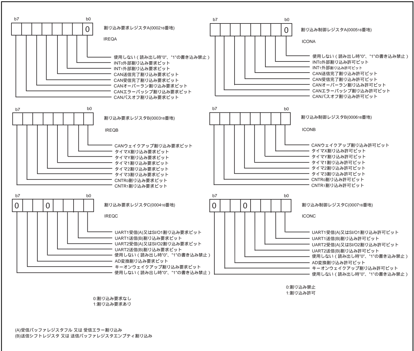
図17. 割り込み関連レジスタ
