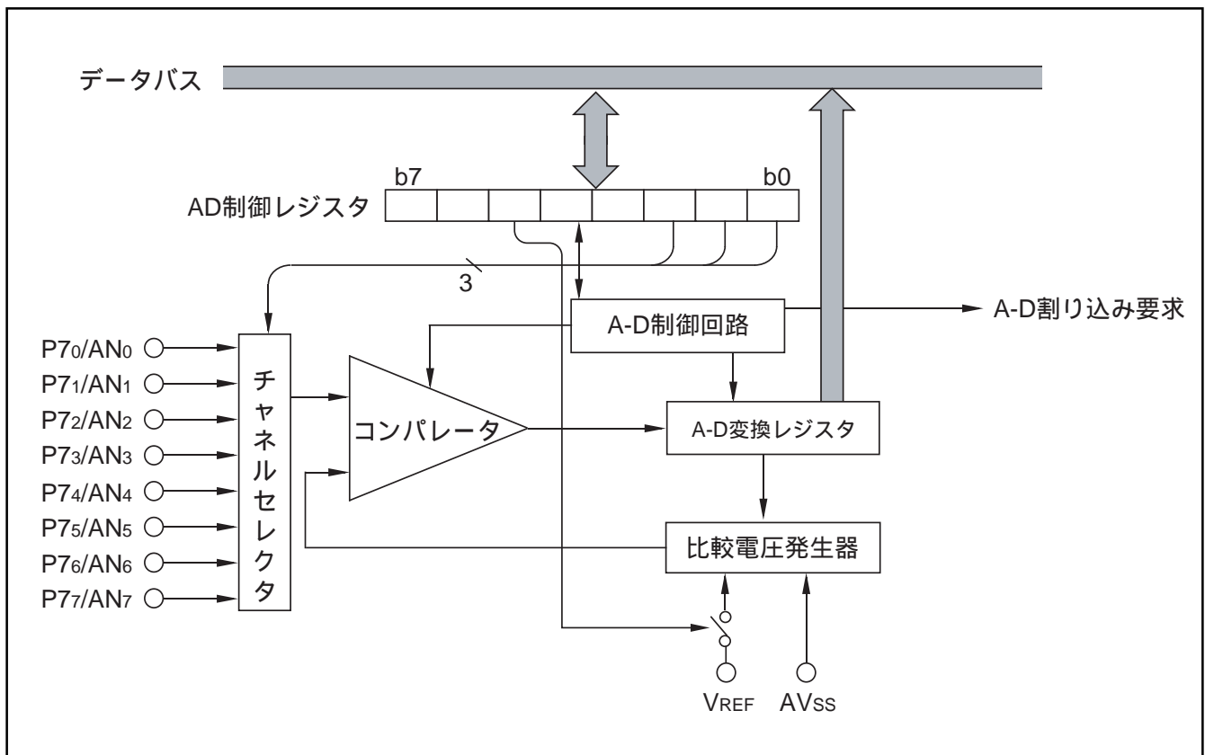
図47. A-D変換器ブロック図
