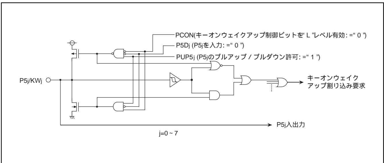
図20. キー入力割り込みブロック図
