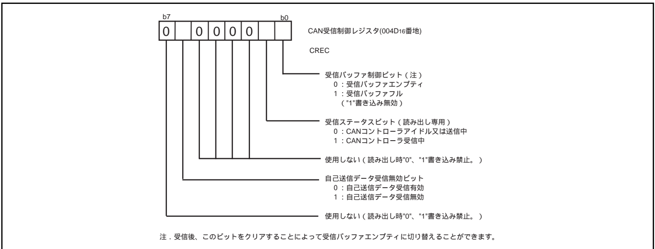
図40. CAN受信制御レジスタ
