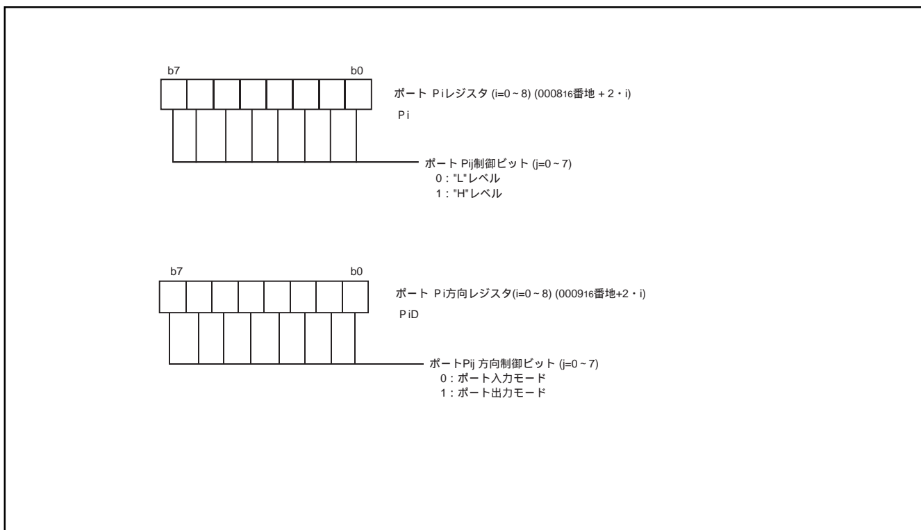
図11. ポート入出力関連レジスタ
