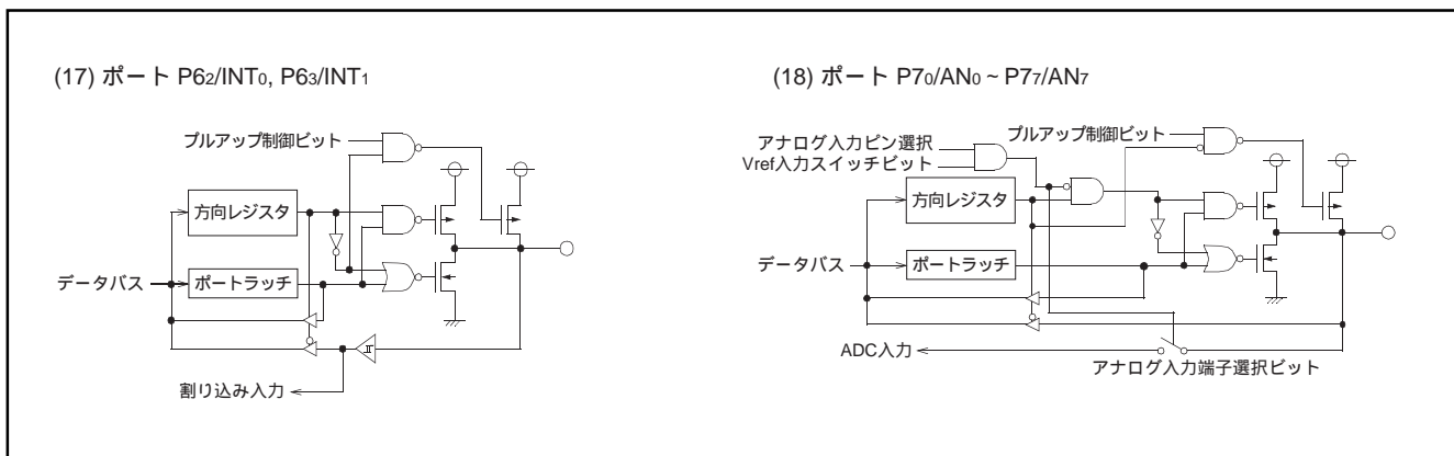
図14. ポートのブロック図(3)
