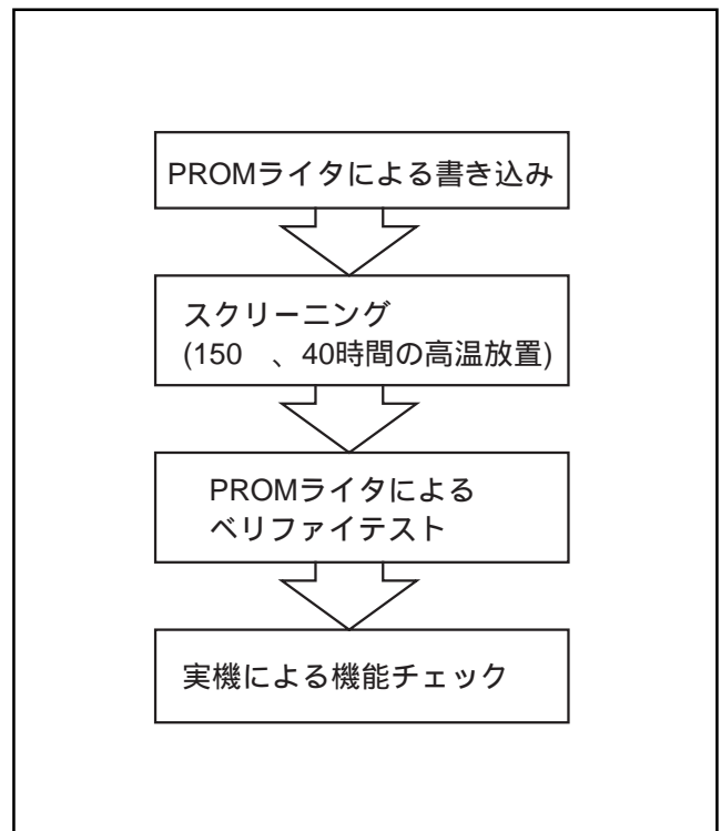
図57. ワンタイムプログラマブル版書き込みとテスト
