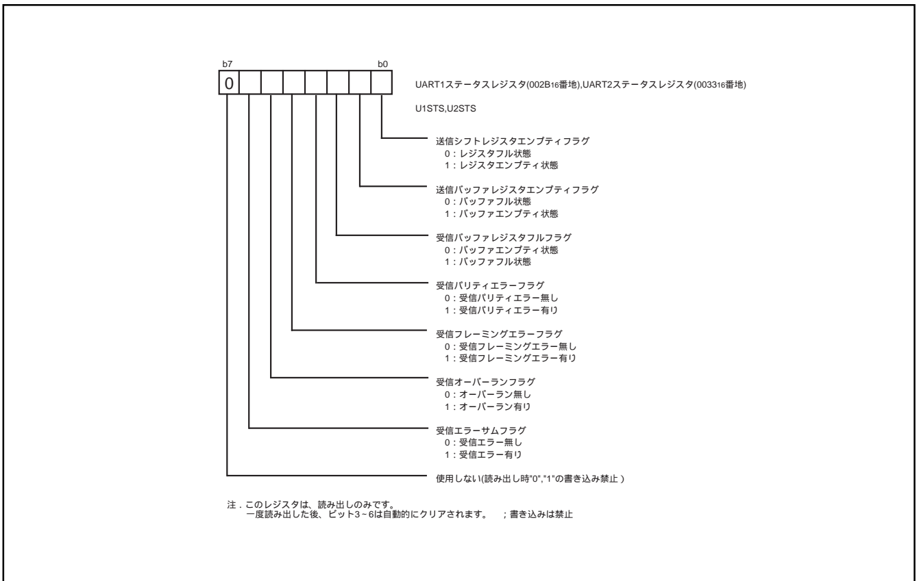
図33. UARTステータスレジスタ
