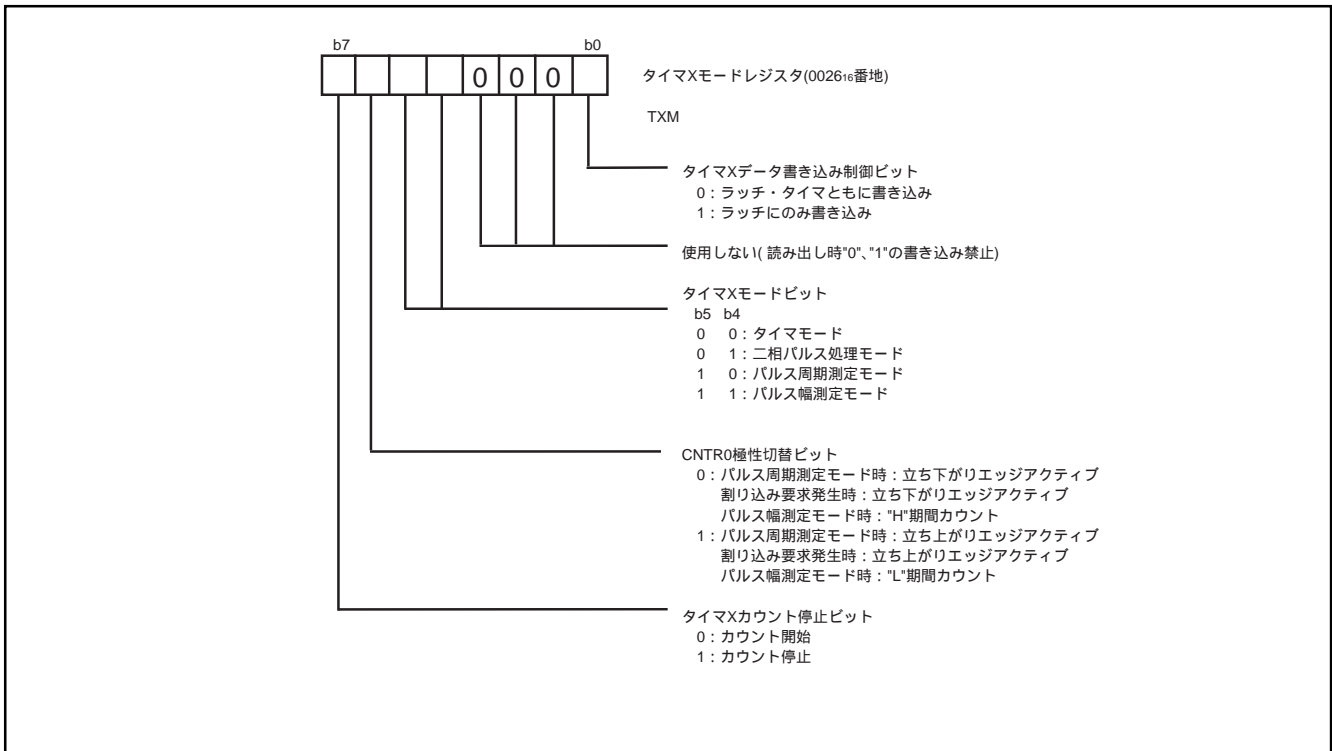
図22. タイマXモードレジスタ
