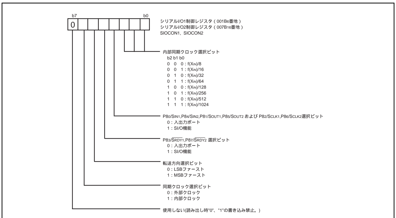
図29. シリアル/O制御レジスタ
