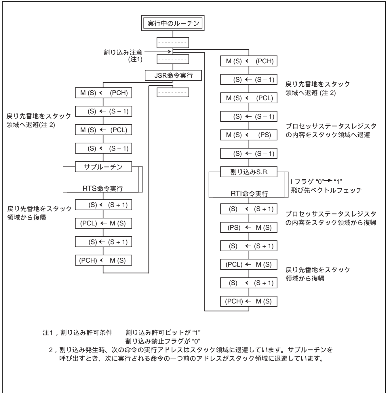
図6. スタックへの退避と復帰動作
