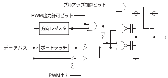
(16) ポート P42/CRX
