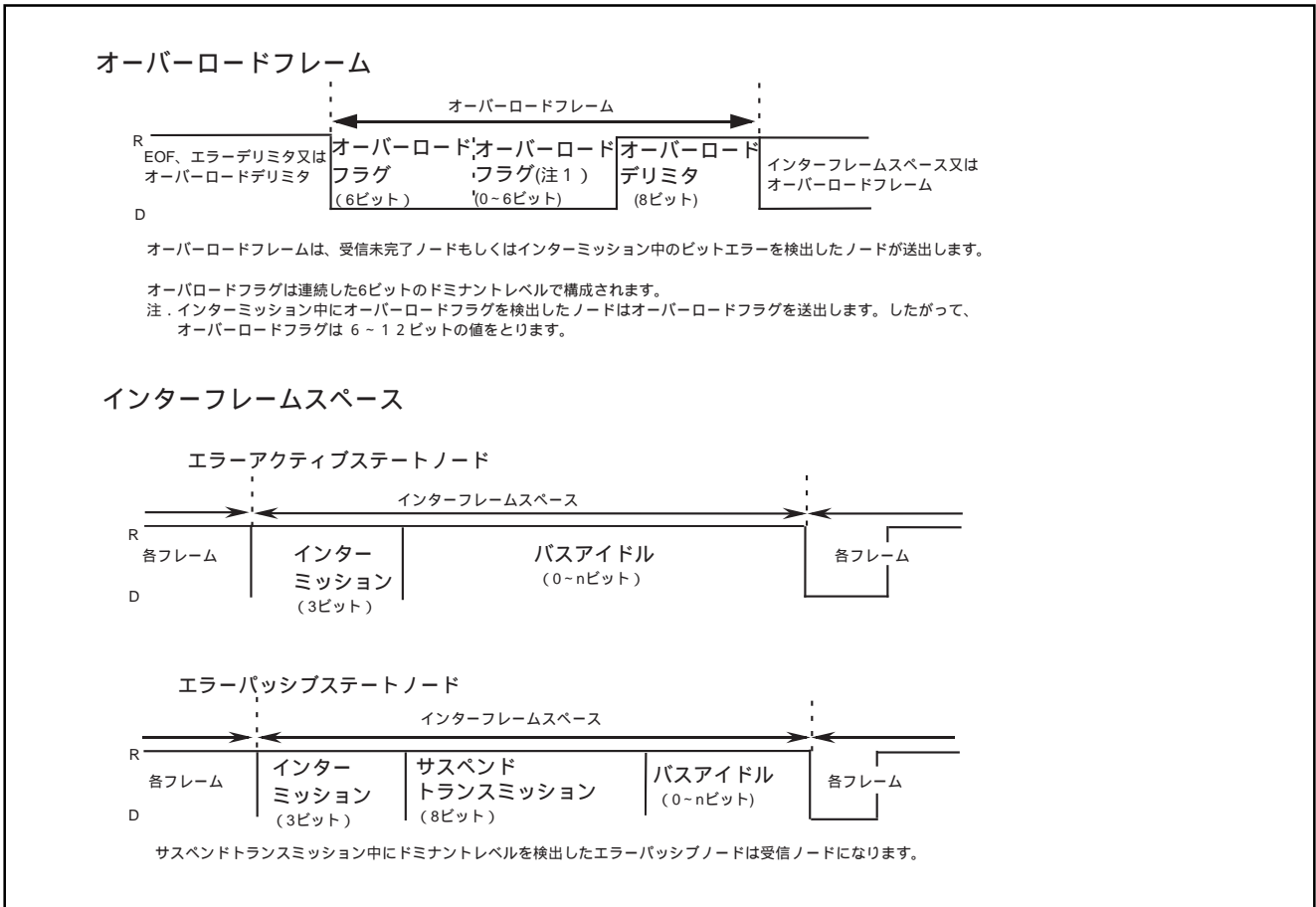
図36. CANプロトコルフレーム 2
