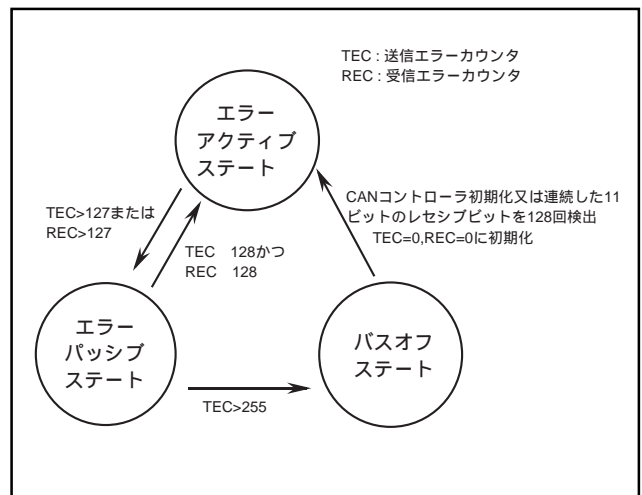
図37. CANコントローラのエラー状態
