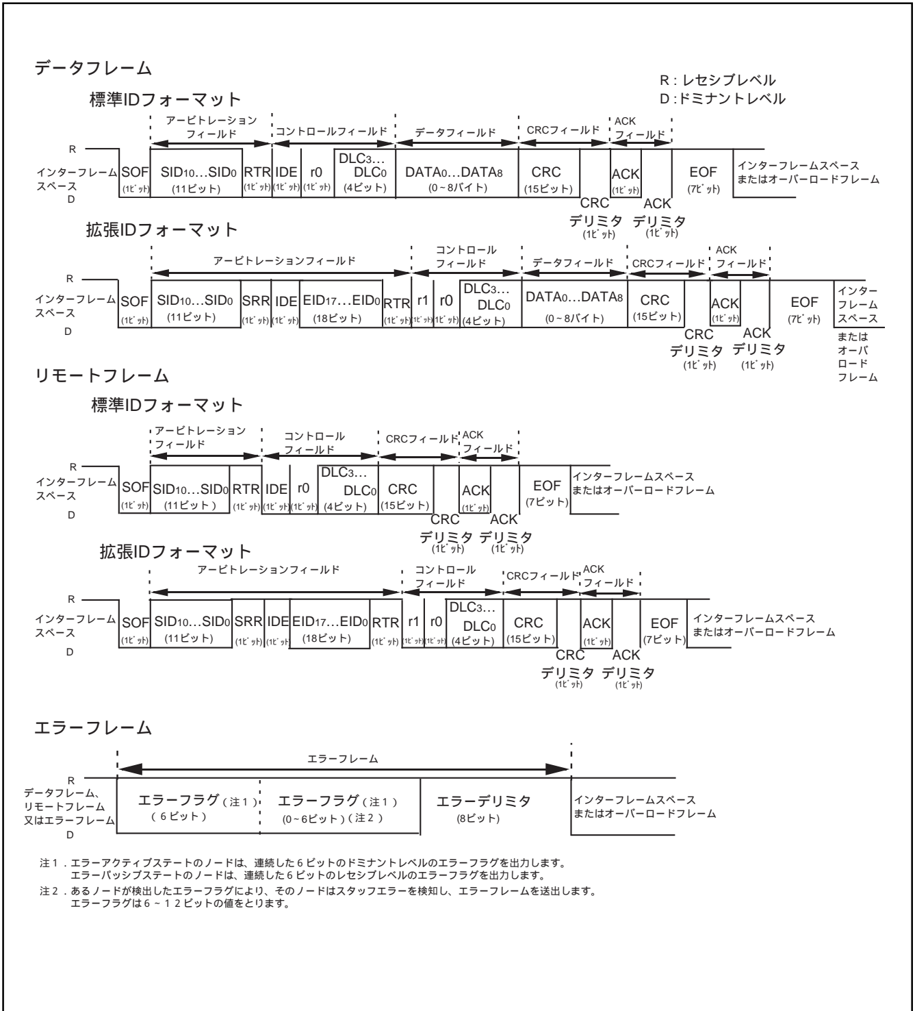
図35. CANプロトコルフレーム 1
