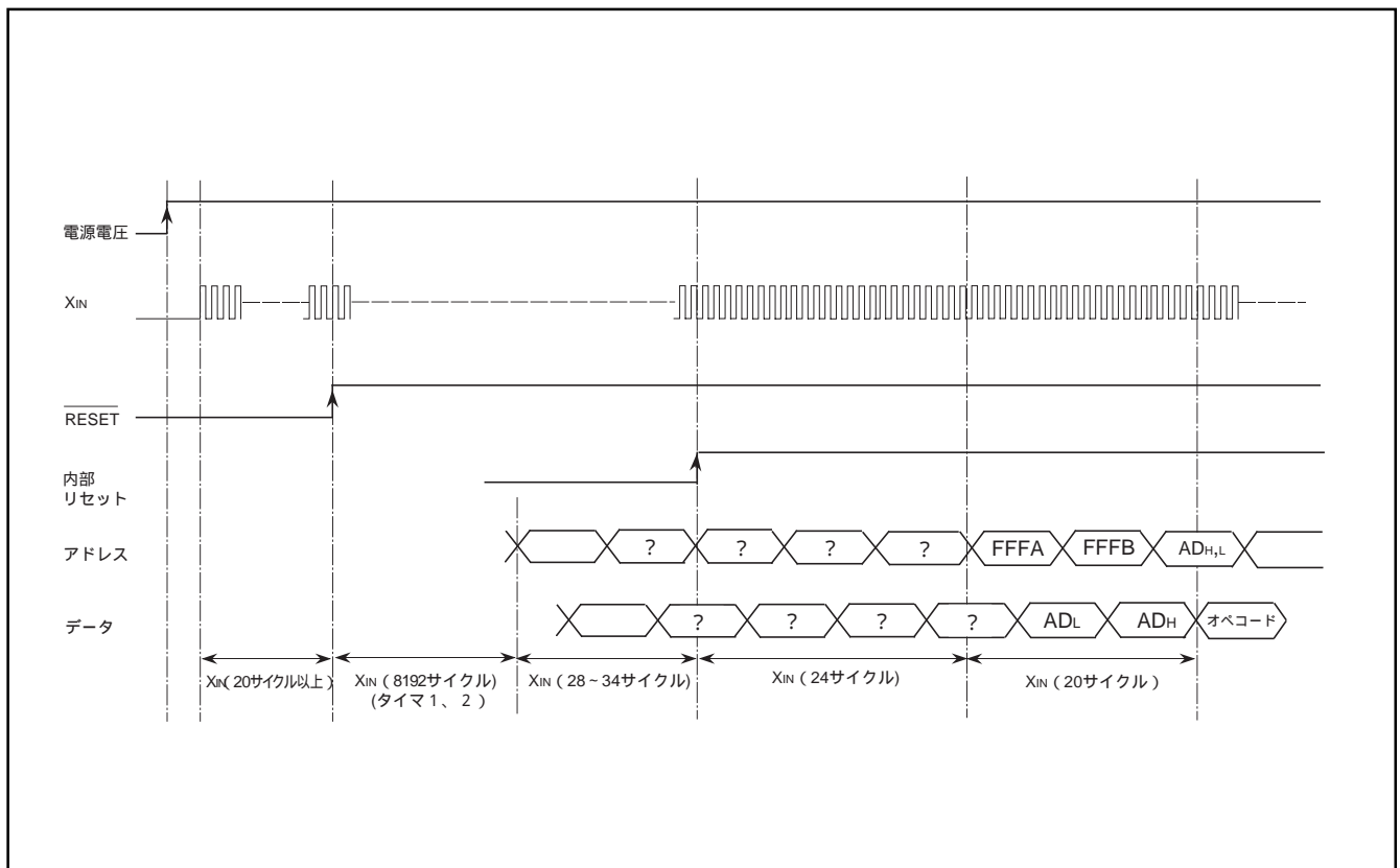
図52. リセットシーケンス
