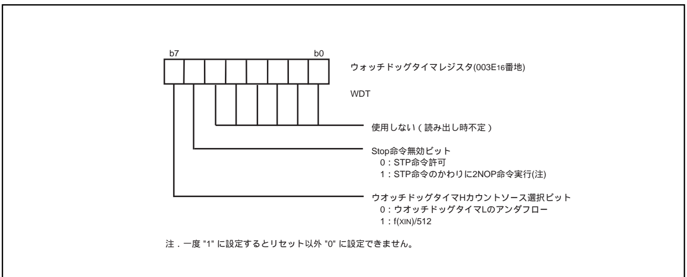
図50. ウォッチドッグタイマレジスタ
