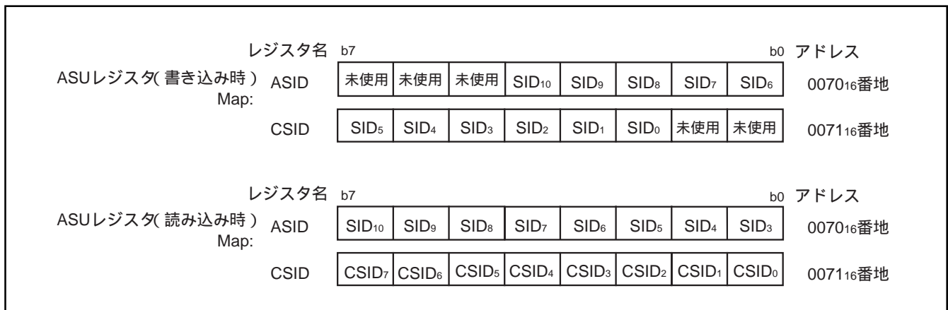
図46. ASUレジスタ
