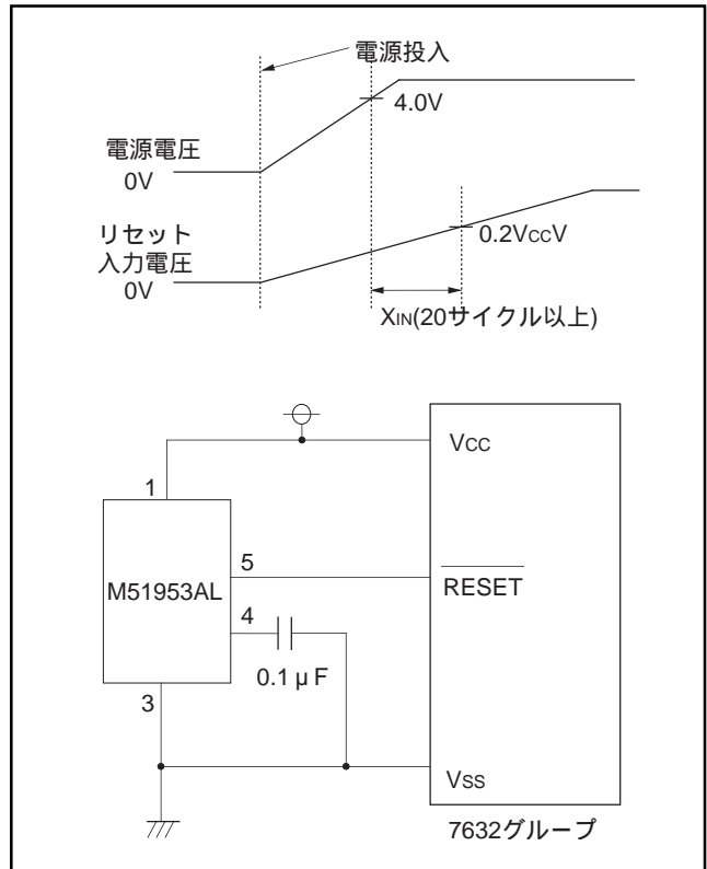
図51. リセット回路例
