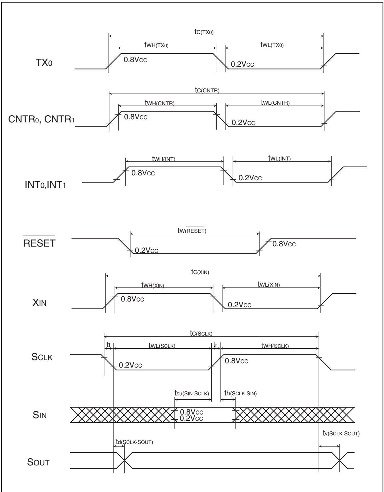
図59. タイミング図
