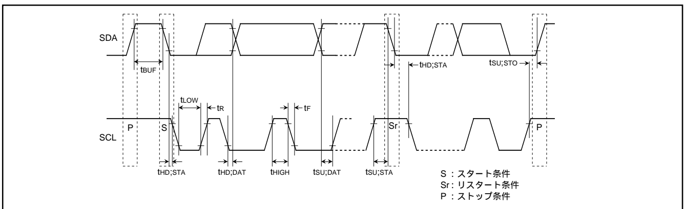
図 14.1 マルチマスタ I 2 C-BUS のタイミング定義図
