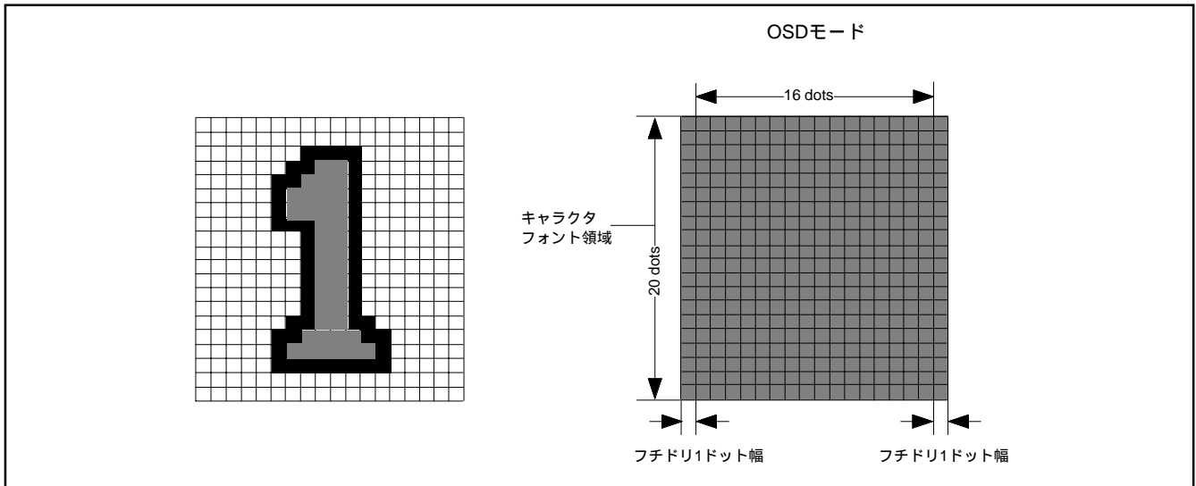
図8.11.20 フチドリ表示例とフチドリ領域
