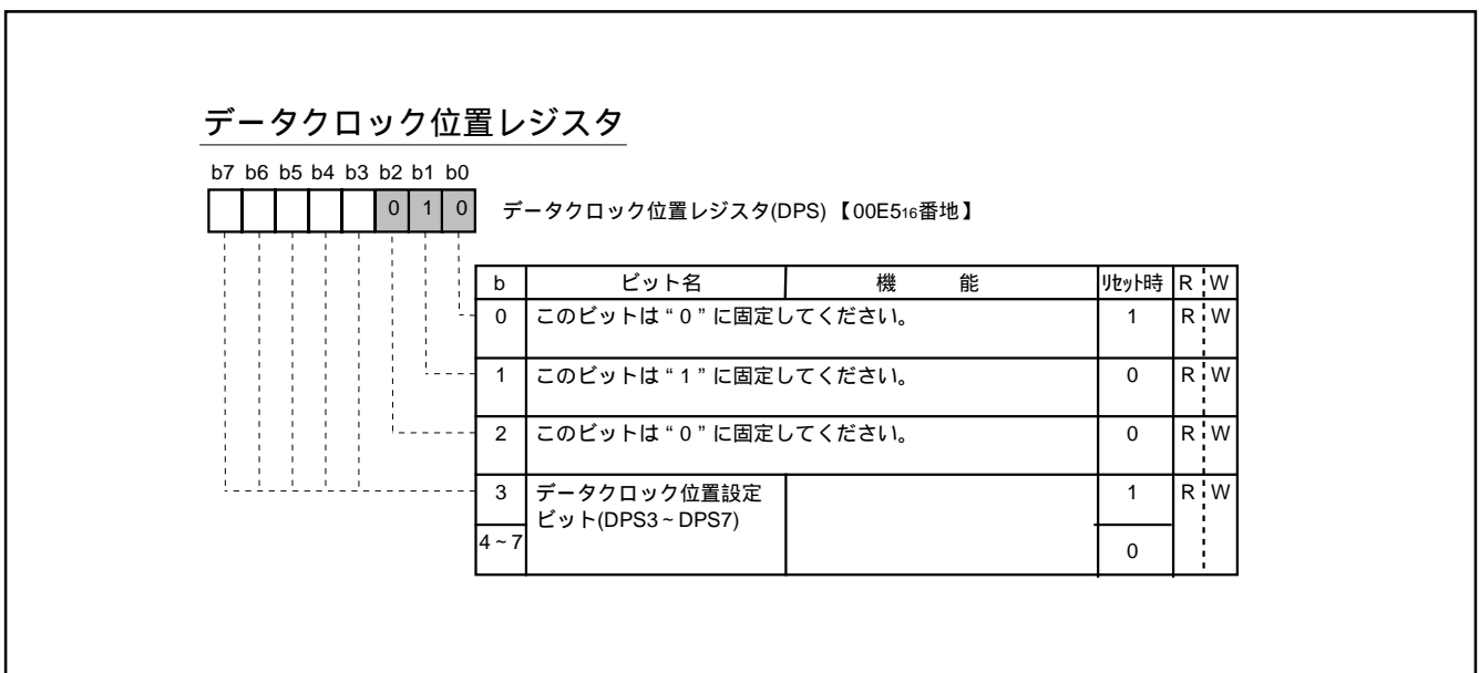
図8.10.11 データクロック位置レジスタ
