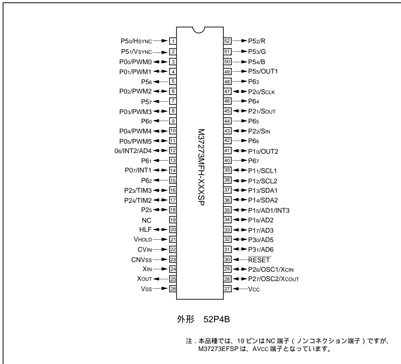
図 4.1 ピン接続図(上面図)
