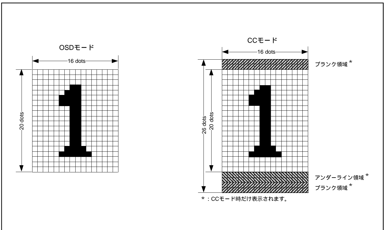
図 8.11.1 OSD 用文字表示領域
