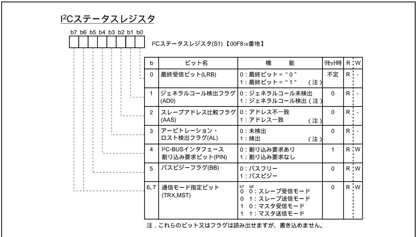
図 8.6.7 I 2 C ステータスレジスタ
