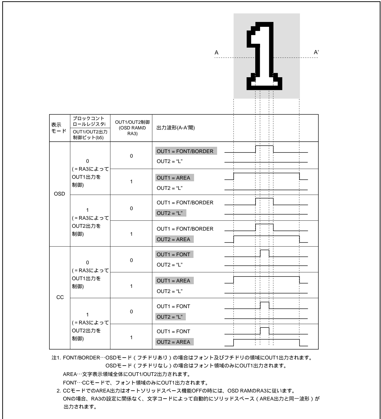
図 8.11.17 OUT1, OUT2 制御の設定値とその波形
