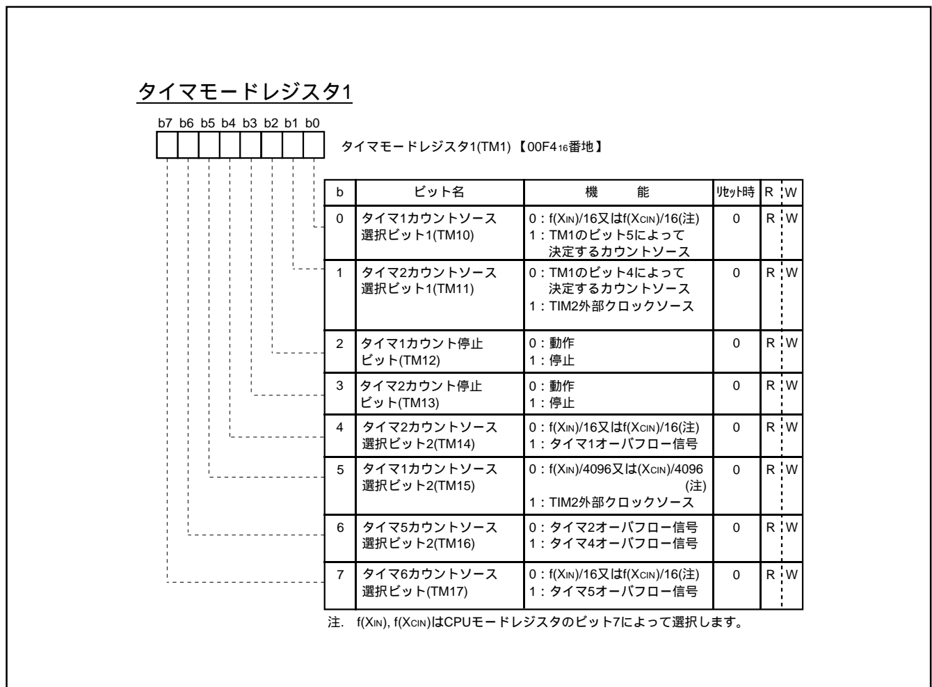
図 8.4.1 タイマモードレジスタ 1
