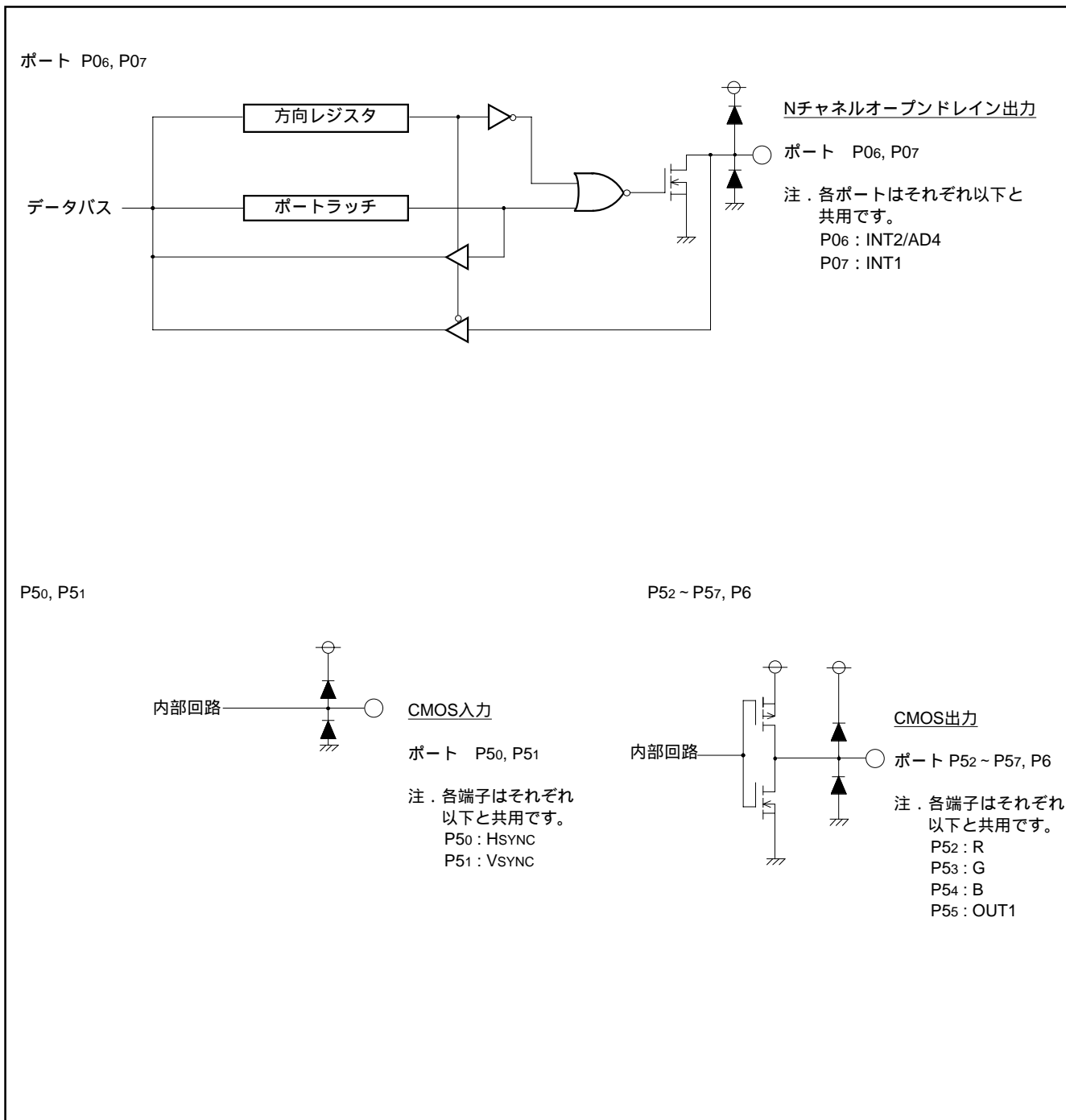
図 7.2 入出力端子のブロック図 (2)
