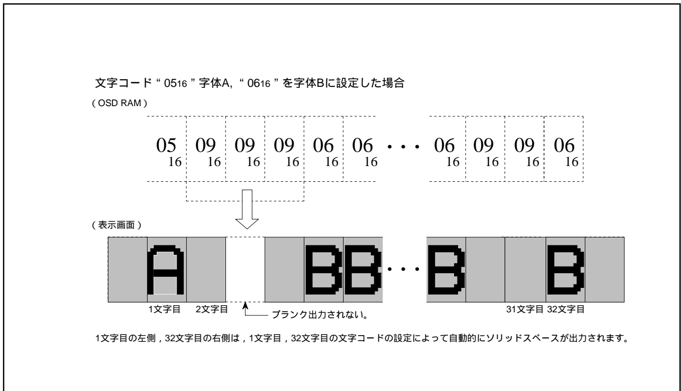
図 8.11.24 オートソリッドスペース画面表示例
