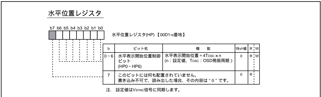
図8.11.8 水平位置レジスタ
