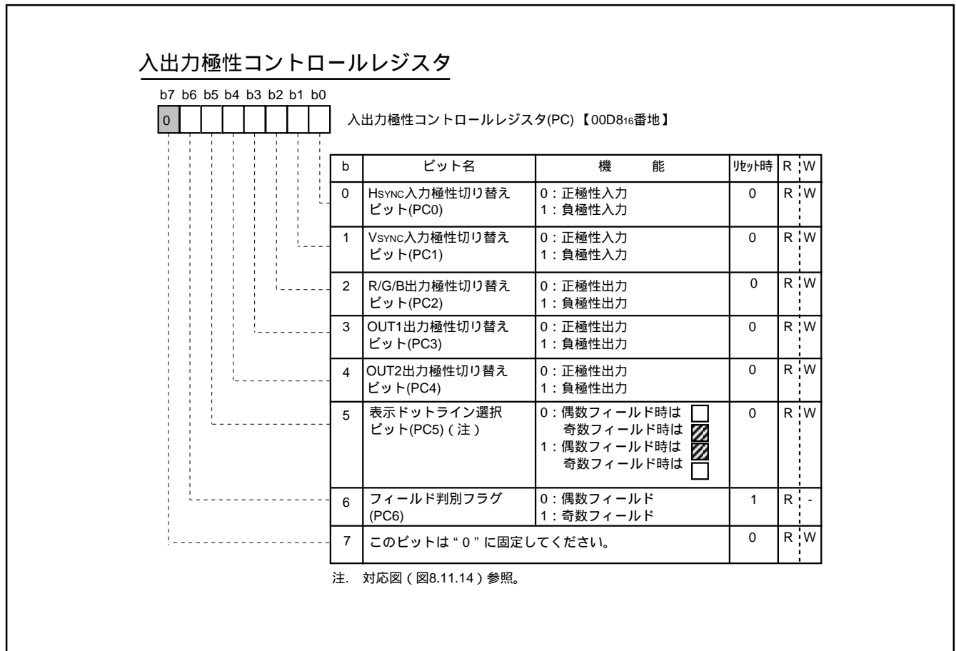
図 8.11.13 入出力極性コントロールレジスタ
