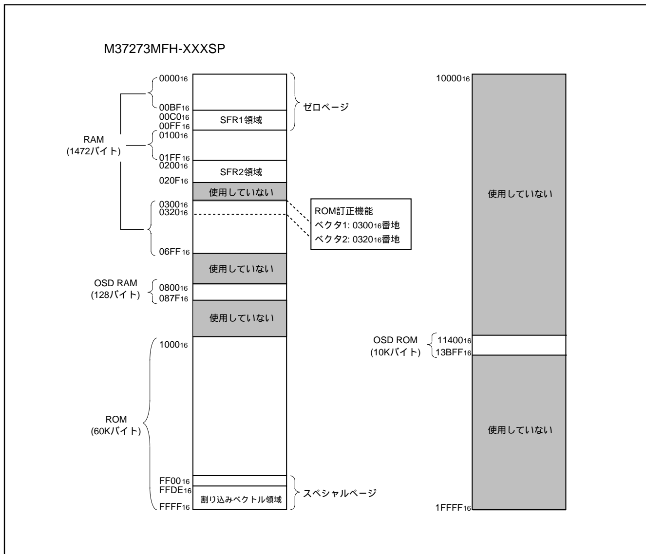
メモリ配置図
