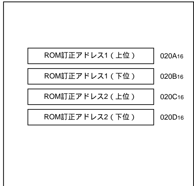
図 8.9.1 ROM 訂正アドレスレジスタ
