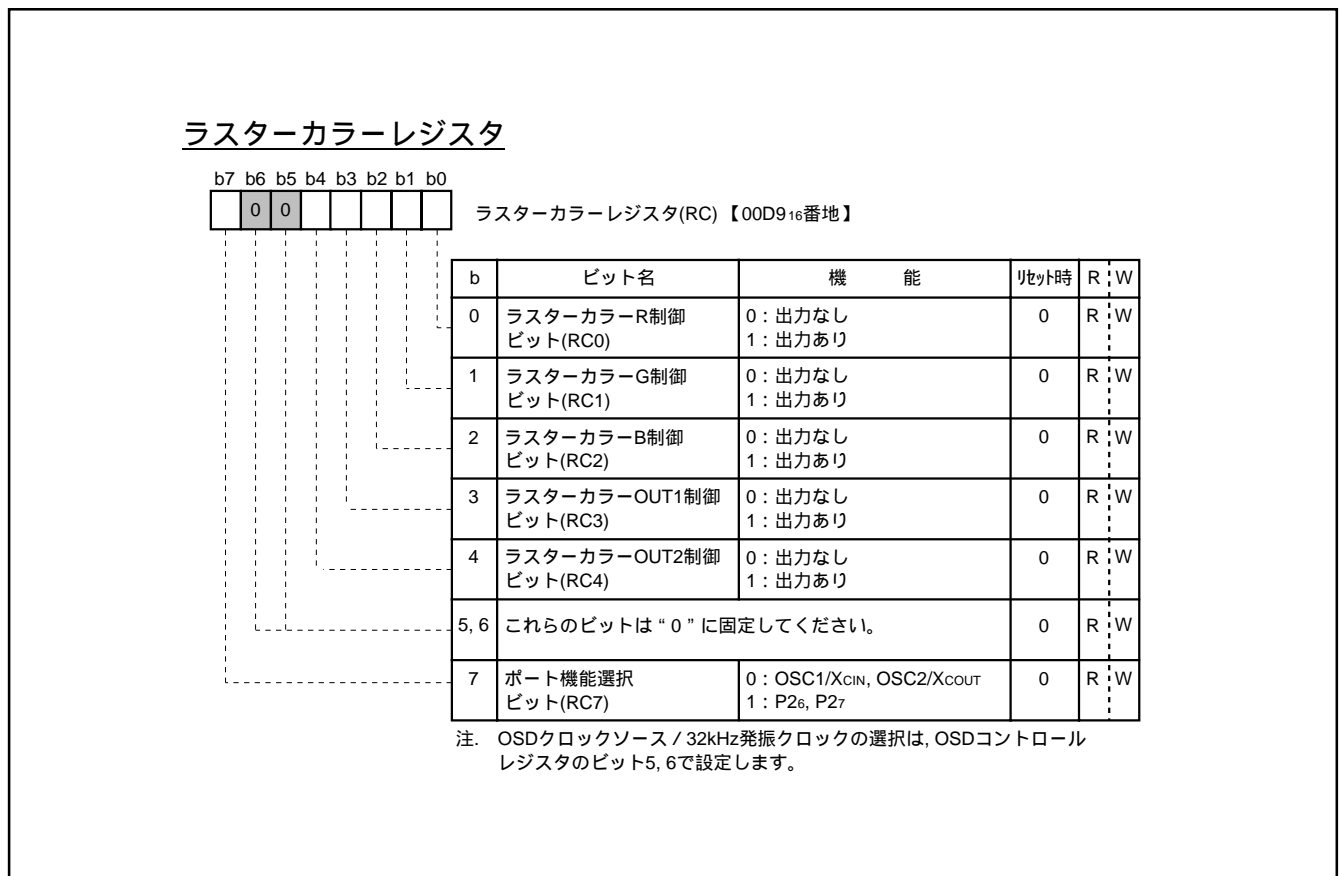
図8.11.29 ラスターカラーレジスタ
