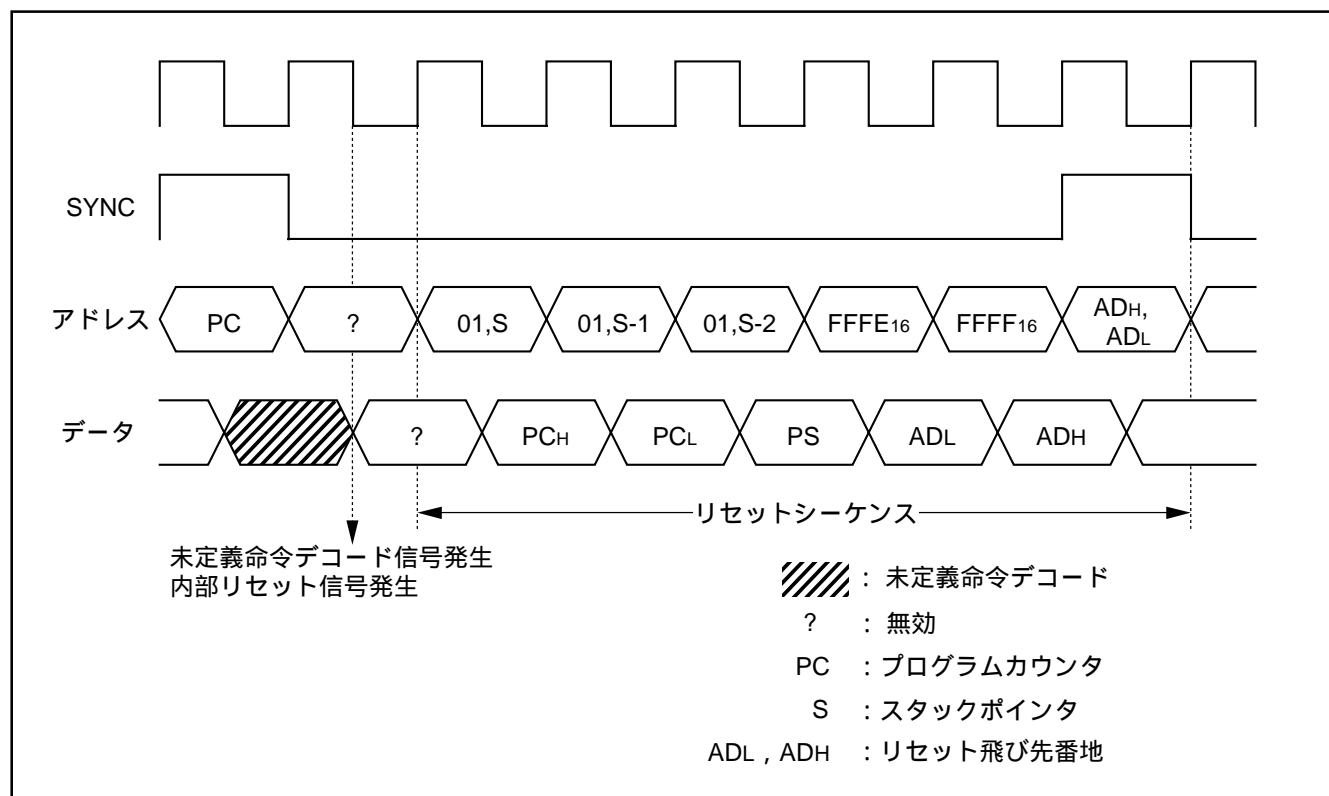
図 8.12.1 暴走検出時のシーケンス
