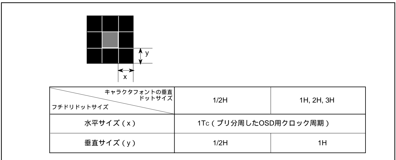
図8.11.21 フチドリの水平サイズ及び垂直サイズ
