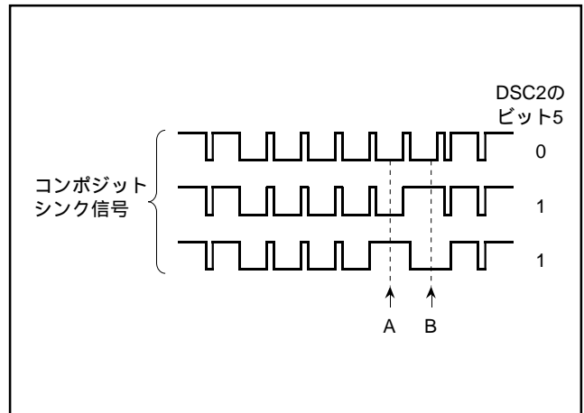
図 8.10.7 Vパルス形状の判別
