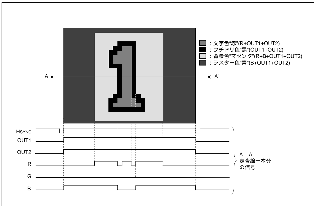
図 8.11.30 ラスター着色例
