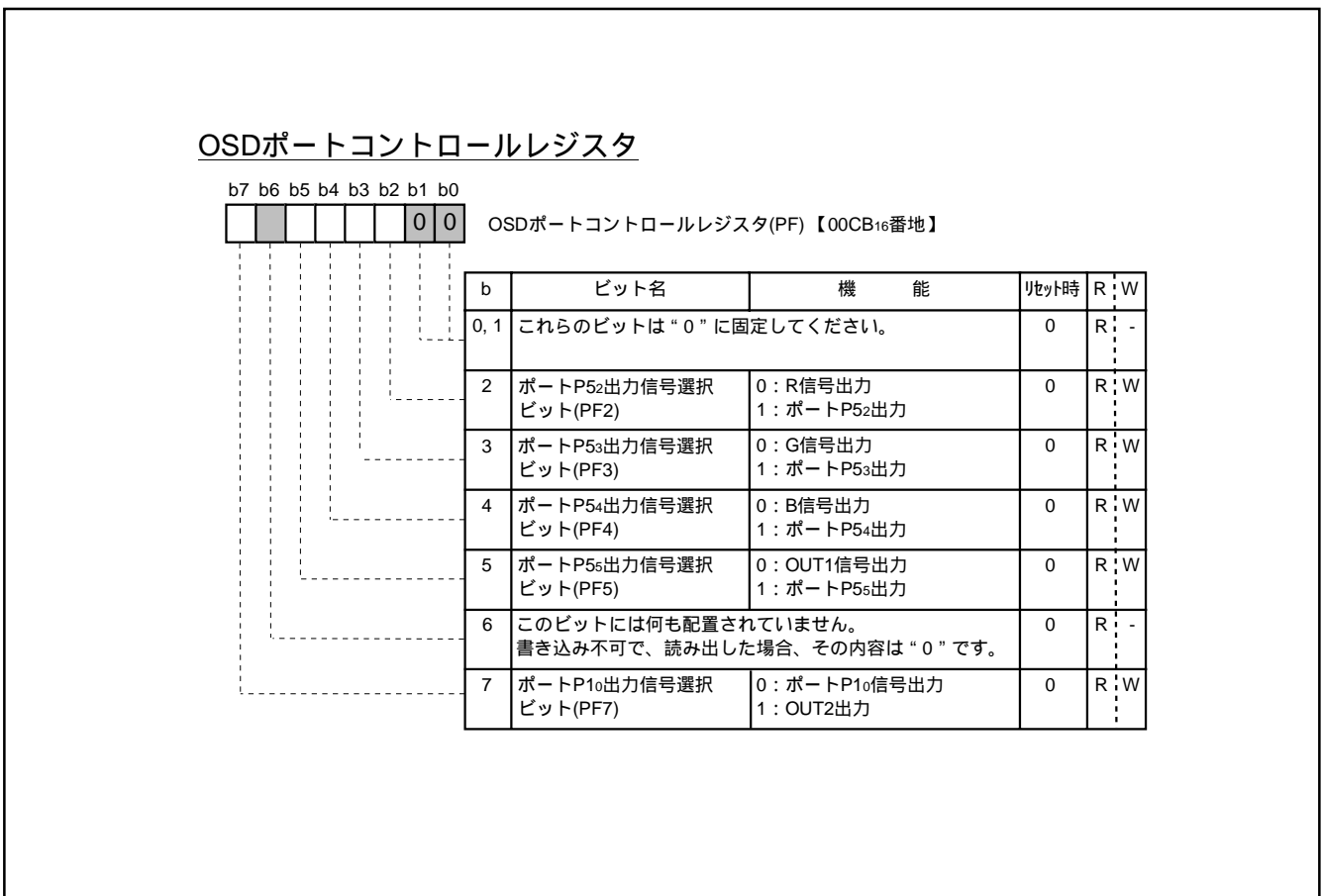
図 8.11.28 OSD ポートコントロールレジスタ
