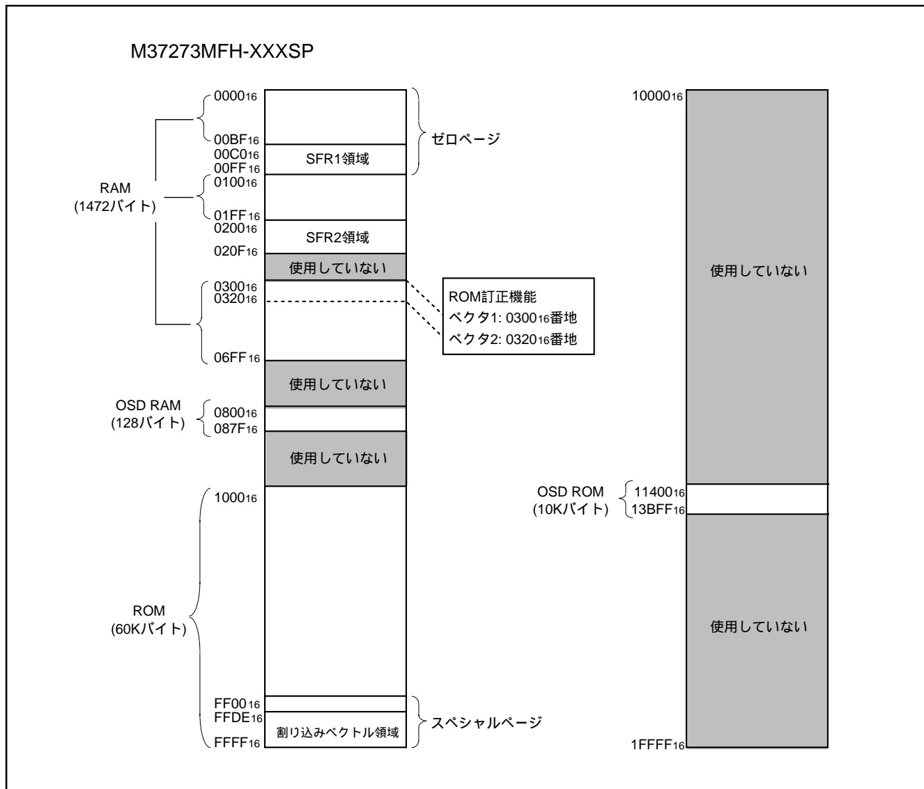
図 8.2.1 メモリ配置図
