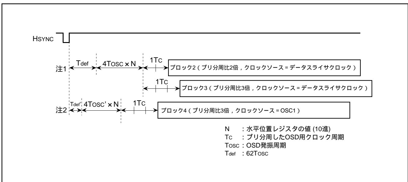
図8.11.9 水平表示開始位置の注意点
