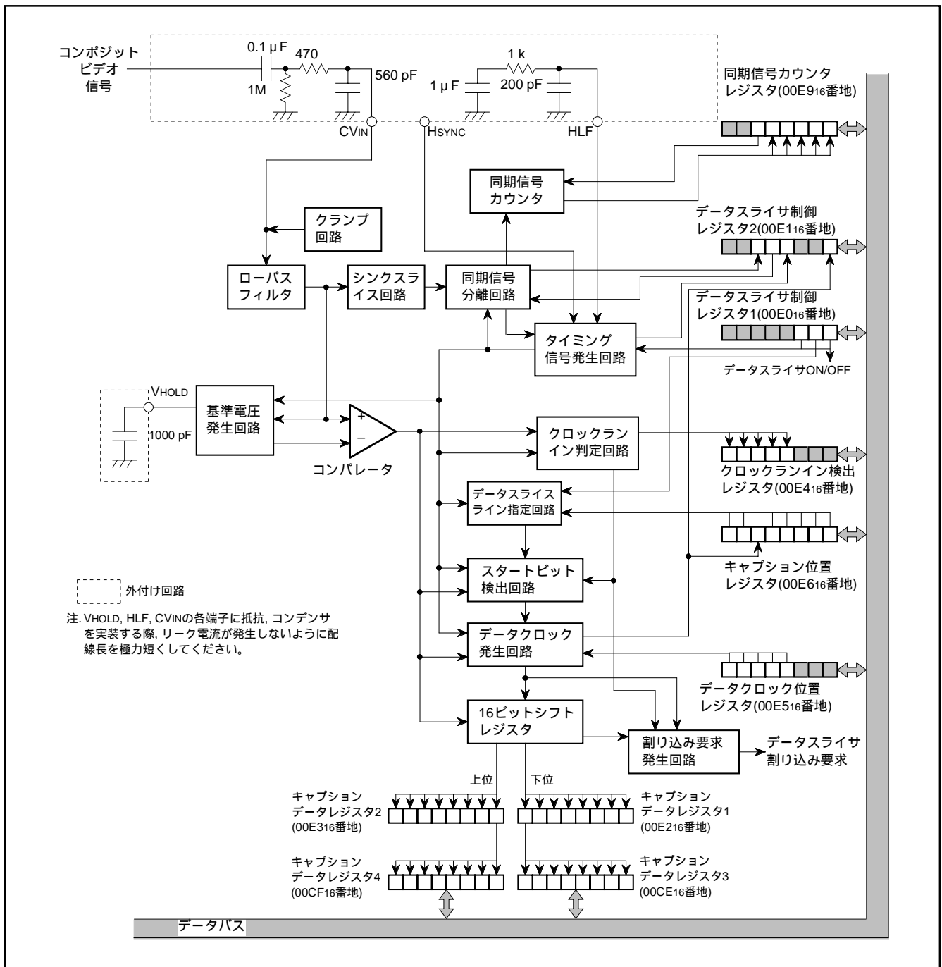
図 8.10.1 データスライサブロック図
