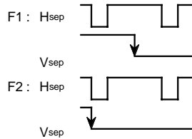
フィールド1 (F1) 及びフィールド2 (F2) の定義
