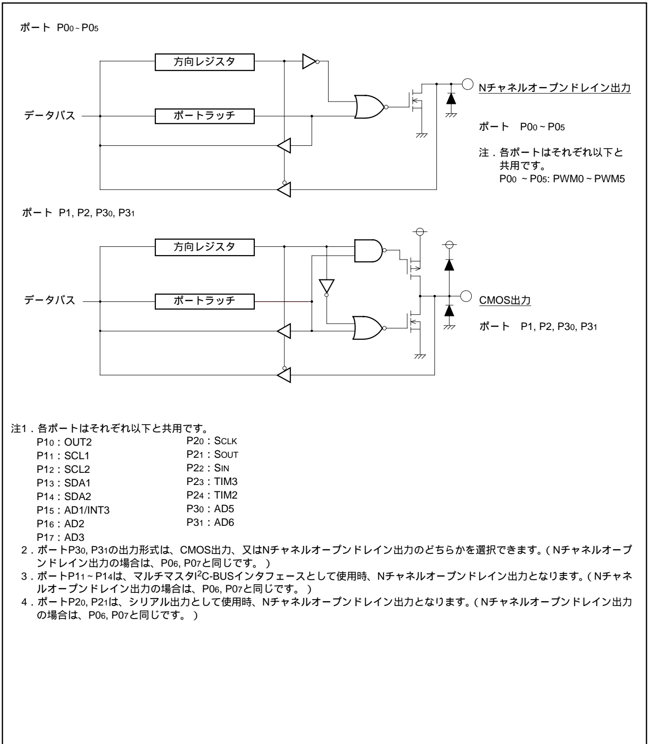
図 7.1 入出力端子のブロック図 (1)
