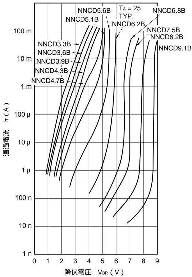
図3 . V BR -I T 特性例 ( 1 )
