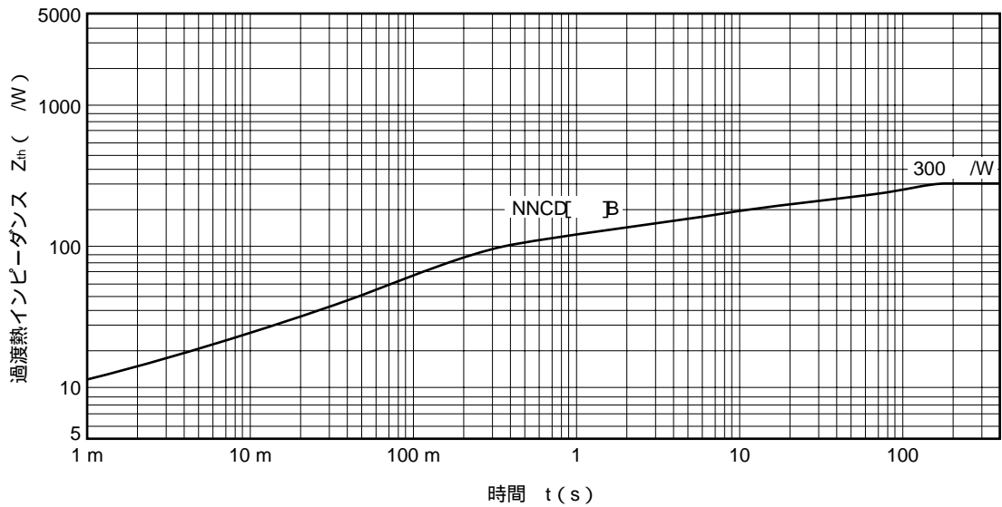
図6 . 過渡熱インピーダンス特性
