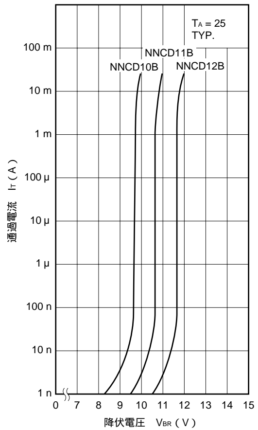
図4 . V BR -I T 特性例 ( 2 )
