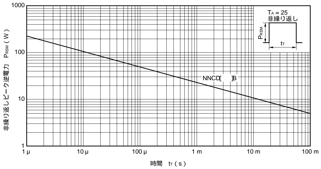
図7. サージ逆電力特性
