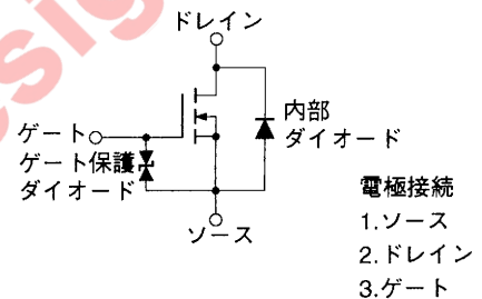
等価回路
