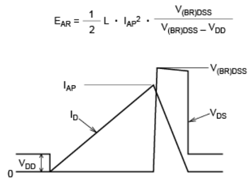
アバランシェ動作波形
