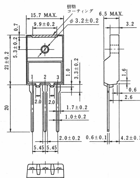
外形図 (単位: mm)
