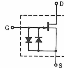
等価接続図
