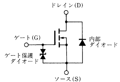
等価回路
