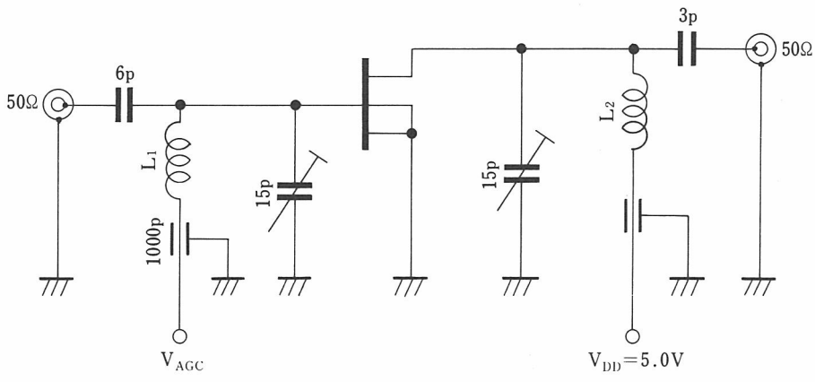
100MHz G_{ps} , NF 測定回路
