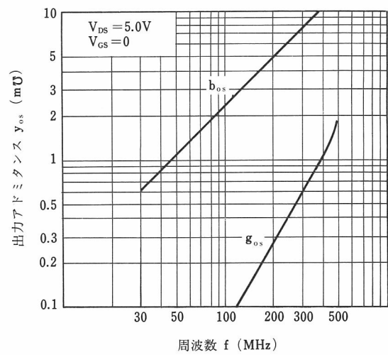
y_{os}-f 特性
