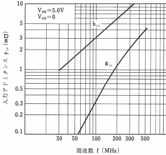
y_{is}-f 特性
