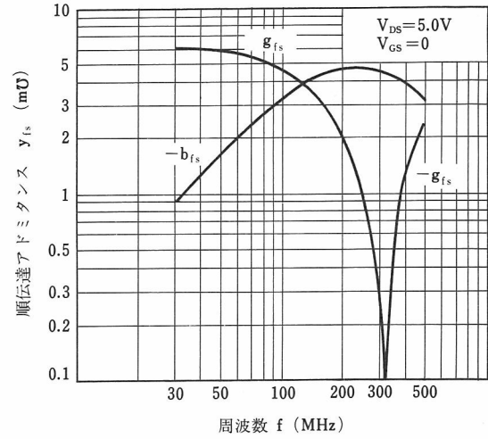
y_{fs}-f 特性
