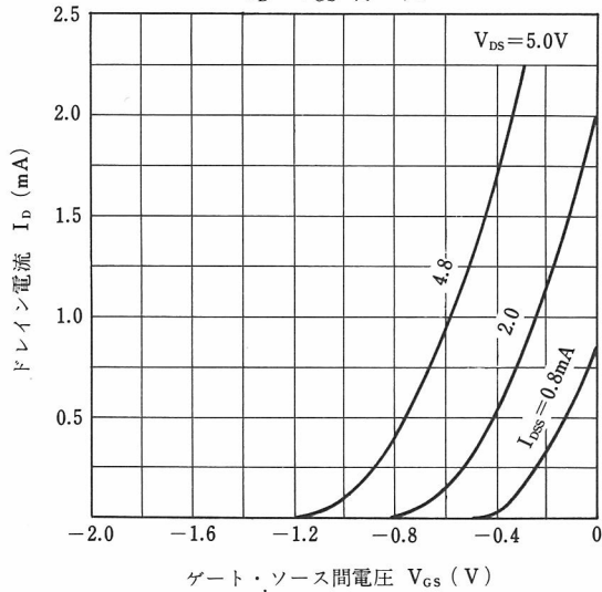
I D -V GS 特性
