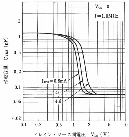
C rss -V DS 特性
