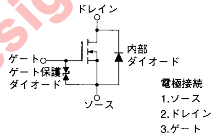
等価回路
