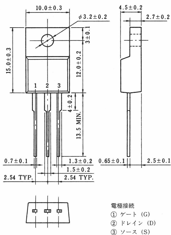
外形図 (単位: mm)
