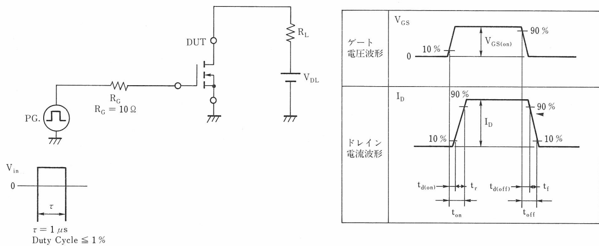
測定回路図 2：スイッチングタイム測定回路
