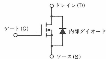
等価回路
