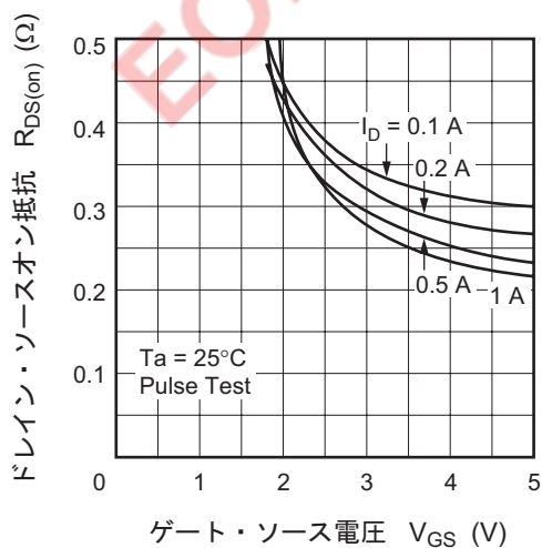
ドレイン・ソースオン抵抗対 ゲート・ソース電圧特性
