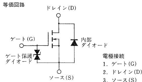
等価回路
