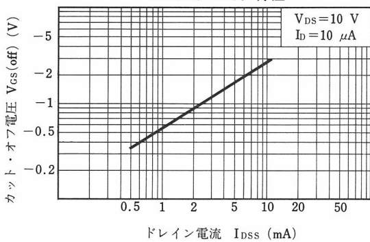
V_{GS(off)} - I_{DSS} 特性
