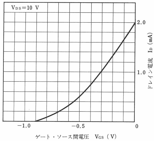
I_D - V_{GS} 特性 ( I_{DSS} = 2.0\text{ mA} )
