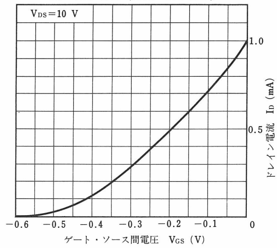
I_D - V_{GS} 特性 ( I_{DSS} = 1.0\text{ mA} )
