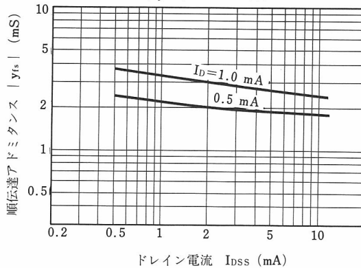
|y_{fs}| - I_{DSS} 特性
