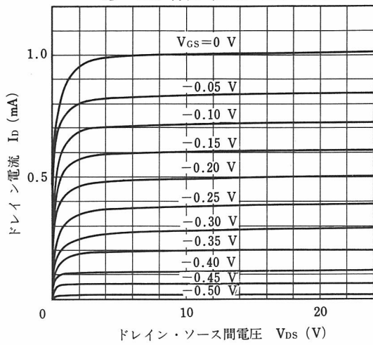
I_D - V_{DS} 特性 ( I_{DSS} = 1.0\text{ mA} )
