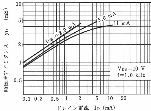
|y_{fs}| - I_D 特性
