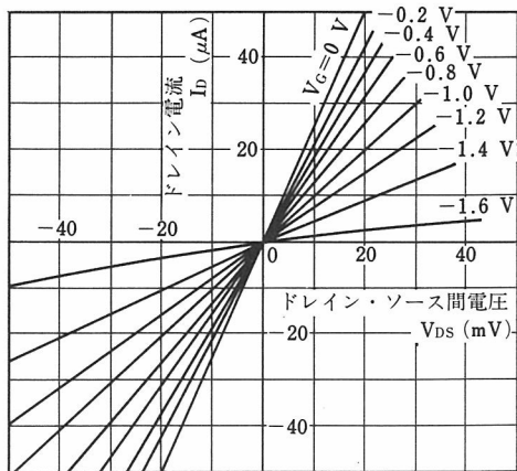
I_D - V_{DS} 特性 ( I_{DSS} = 5.0 \text{ mA} )
