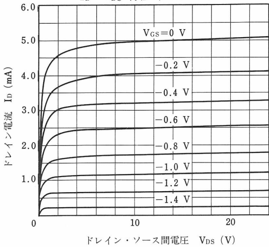
I_D - V_{DS} 特性 ( I_{DSS} = 5.0\text{ mA} )
