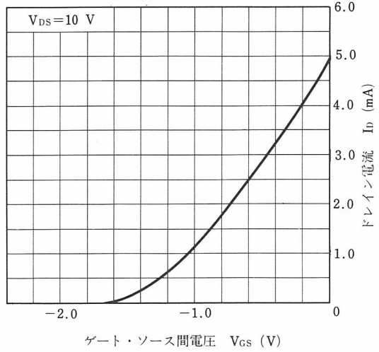
I_D - V_{GS} 特性 ( I_{DSS} = 5.0\text{ mA} )
