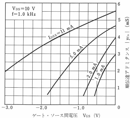
|y_{fs}| - V_{GS} 特性
