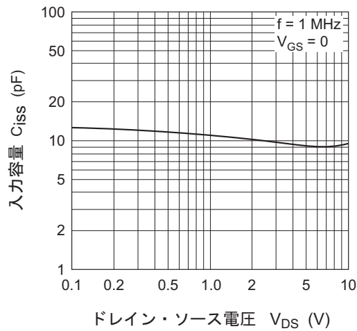
入力容量対ドレイン・ソース電圧特性
