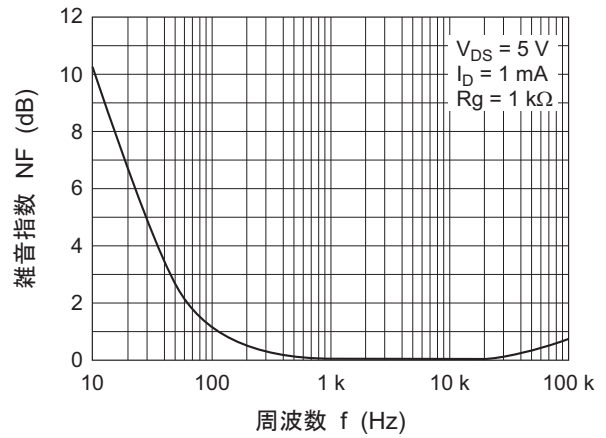
雑音指数対周波数
