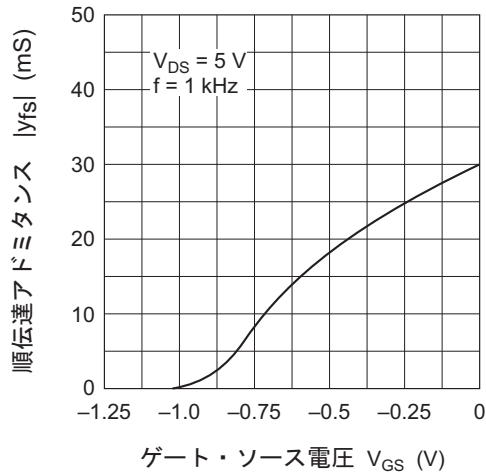
順伝達アドミタンス対 ゲート・ソース電圧
