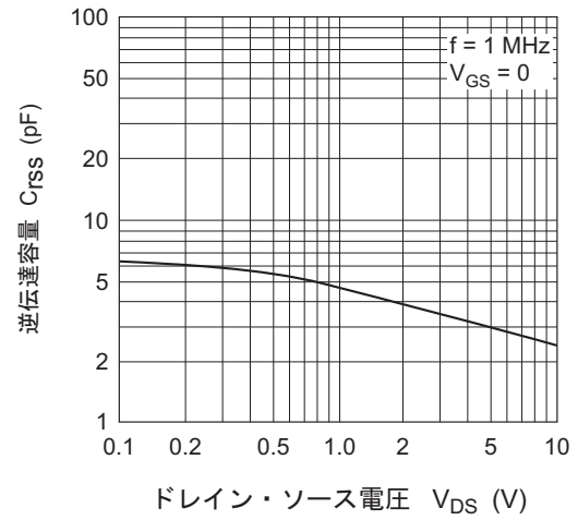
逆伝達容量対 ドレイン・ソース電圧
