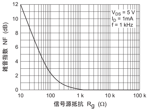
雑音指数対信号源抵抗
