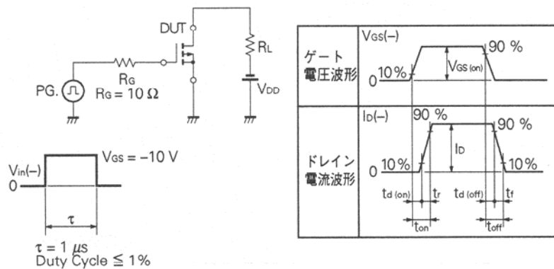
測定回路図 1 : スイッチングタイム測定回路
