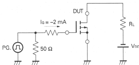
測定回路図 2 : ゲート電荷量測定回路
