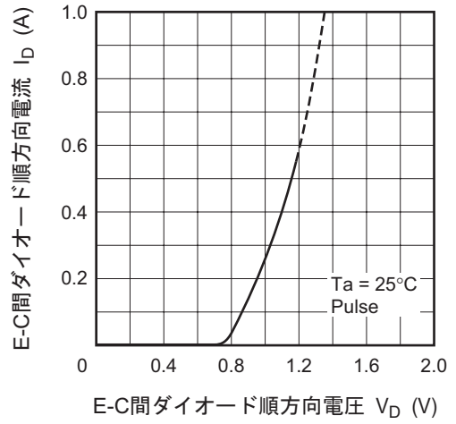
E-C間ダイオード特性
