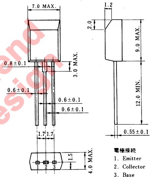
外形図 (Unit: mm)
