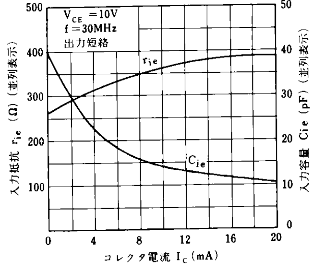
r_{ie}, C_{ie} - I_C 特性
