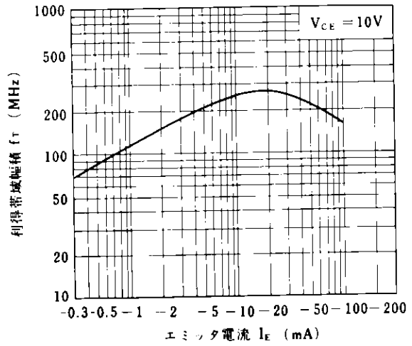
f_T - I_E 特性
