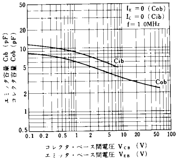
C_{ib} - V_{EB} , C_{ob} - V_{CB} 特性
