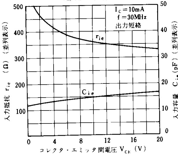
r_{ie}, C_{ie} - V_{CE} 特性
