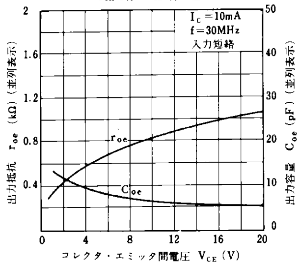
r_{oe}, C_{oe}-V_{CE} 特性
