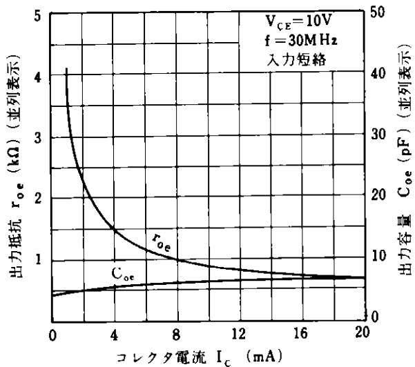
r_{oe}, C_{oe}-I_C 特性
