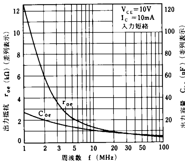
r_{oe}, C_{oe}-f 特性
