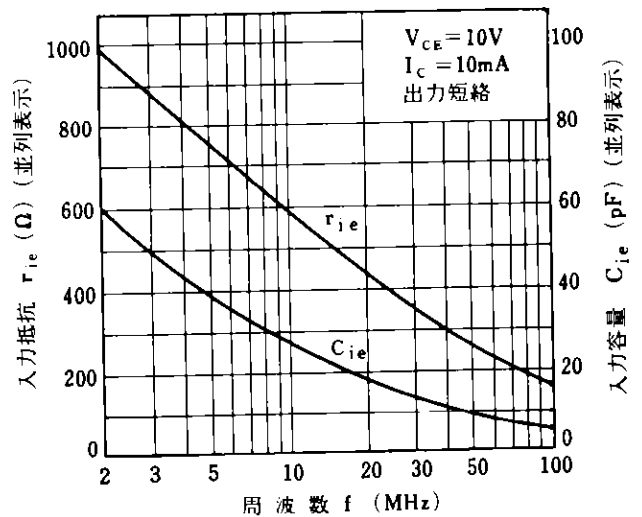
r_{ie}, C_{ie} - f 特性
