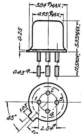
外形図 (単位 mm) NDS-TX-4
