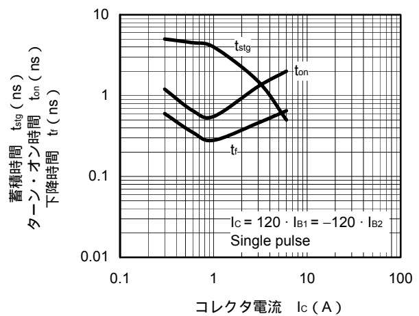
SW - I_c 特性
