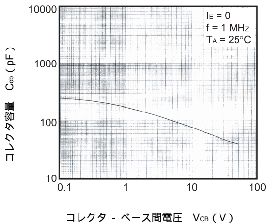
C_{ob} - V_{CB} 特性
