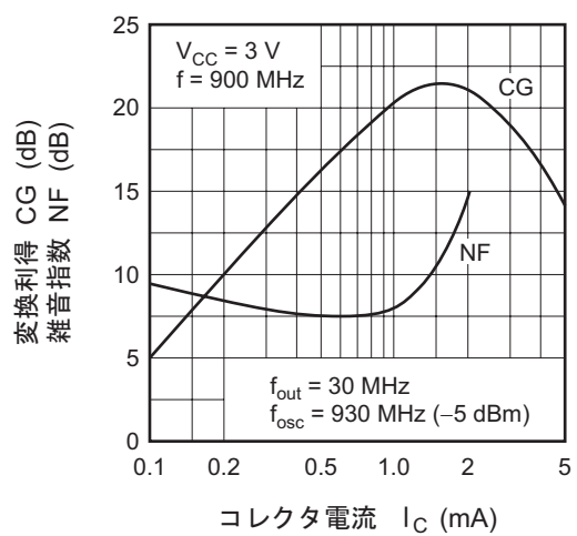
変換利得, 雑音指数対コレクタ電流特性
