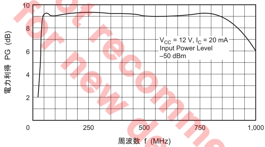
電力利得対周波数特性
