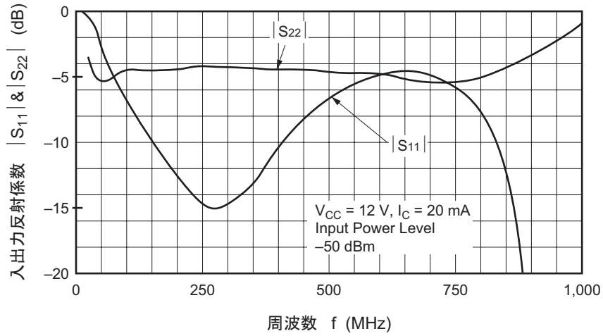
入出力反射係数対周波数
