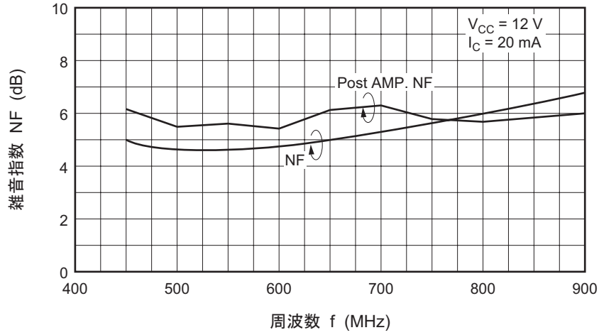
雑音指数対周波数特性
