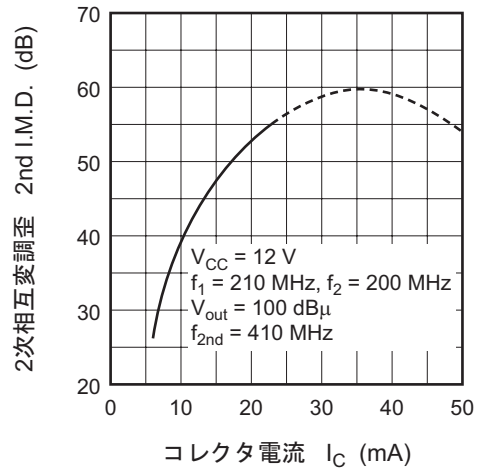
2次相互変調歪対コレクタ電流特性
