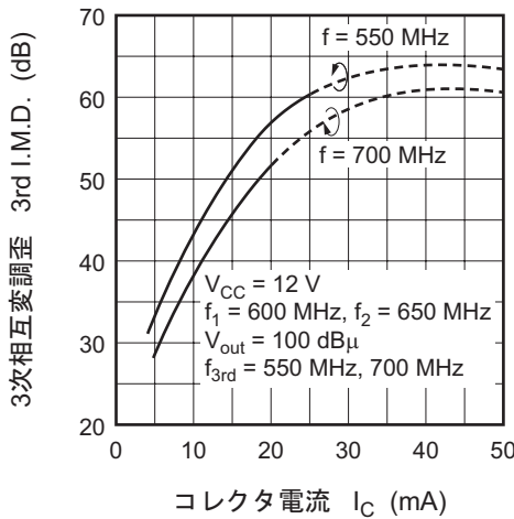
3次相互変調歪対コレクタ電流特性
