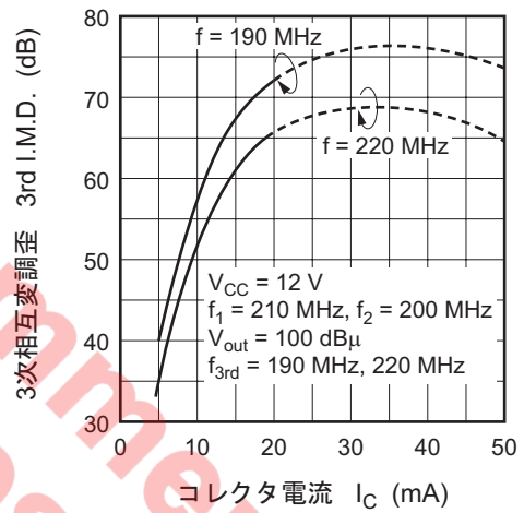
3次相互変調歪対コレクタ電流特性
