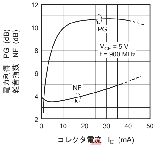
電力利得・雑音指数対コレクタ電流特性
