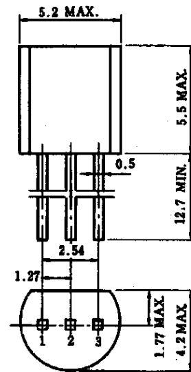
外形図(Unit: mm)
