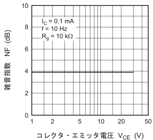
雑音指数対 コレクタ・エミッタ電圧特性
