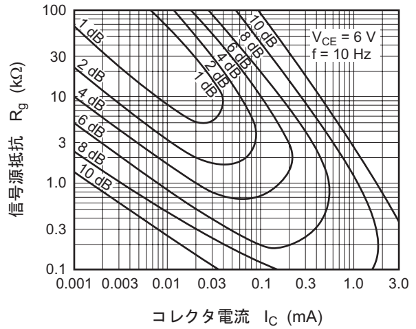
雑音特性
