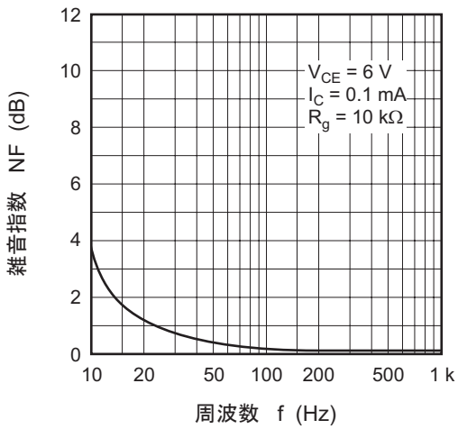
雑音指数対周波数特性
