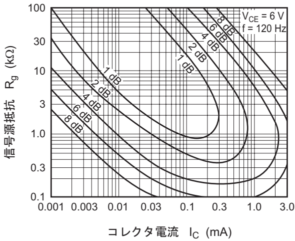
雑音特性
