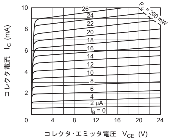
エミッタ接地出力静特性
