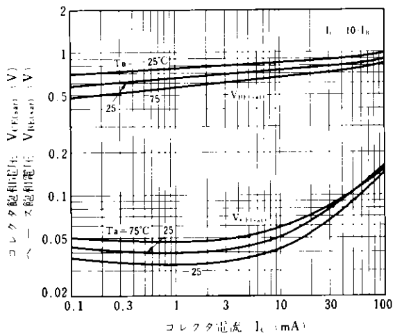
V_{CE(sat)}, V_{BE(sat)} - I_C 特性
