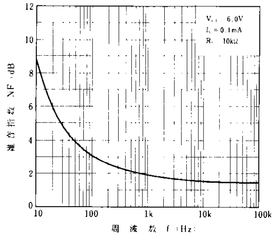
NF - f 特性
