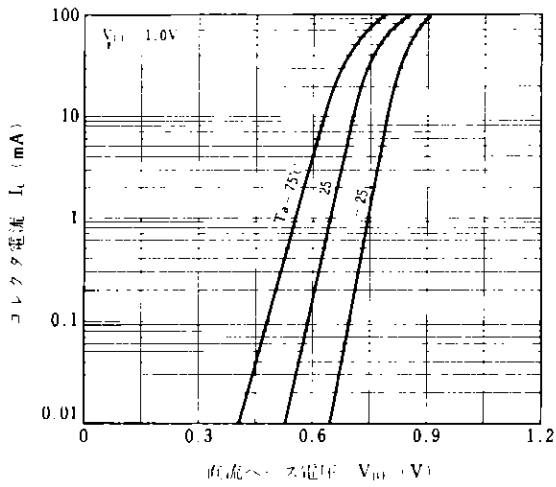
I_C - V_{BE} 特性
