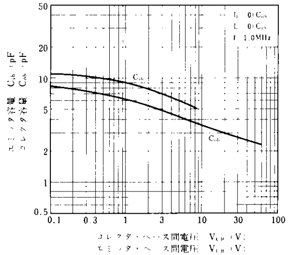
C_{ob} - V_{CB} 特性 C_{ib} - V_{EB}
