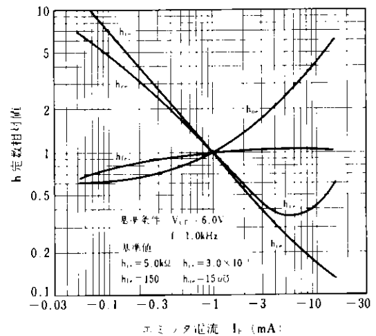
h 定数相対値 - I_E 特性
