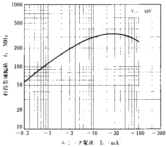
f_T - I_E 特性
