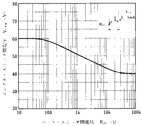
V_{CE} - R_{BE} 特性
