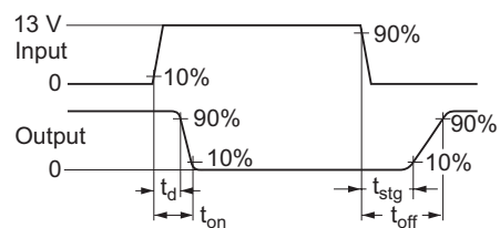
応答波形
