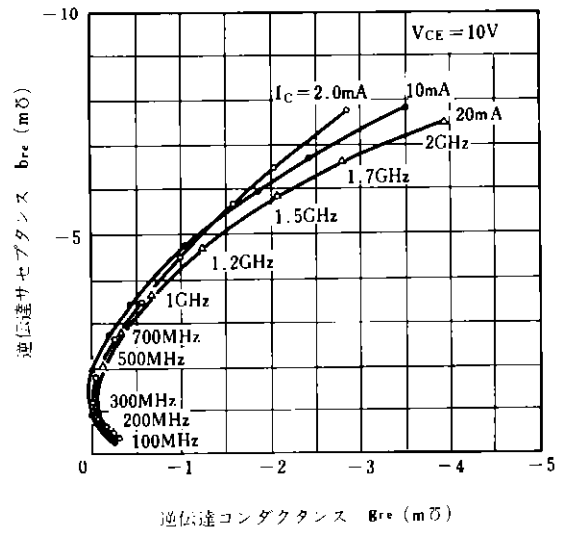
y_{re}-f 特性
