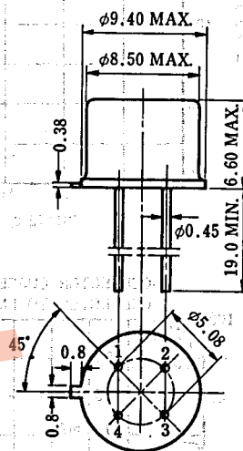
外形図 (単位: mm)
