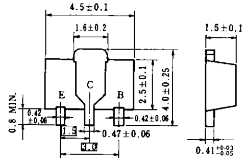
外形図 (単位: mm)
