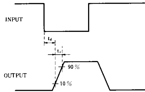
電圧波形
