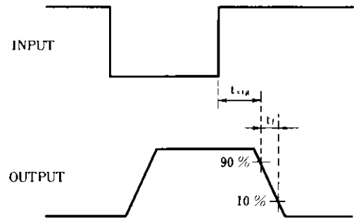
電圧波形
