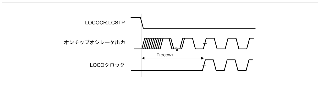
図 2.28 LOCO クロック発振開始タイミング
