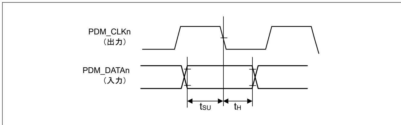
図 2.126 受信タイミング (PDM_CLKn の立ち下がりに同期)
