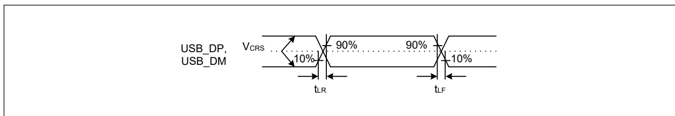
図 2.127 Low-speed モードにおける USB_DP、USB_DM の出力タイミング
