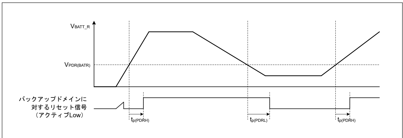
図 2.151 バックアップドメインリセット特性
