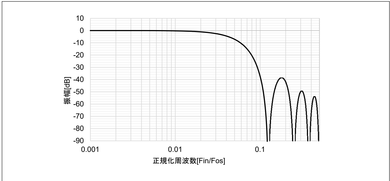
図 2.139 デジタルフィルタ特性 (Sinc フィルタ)
