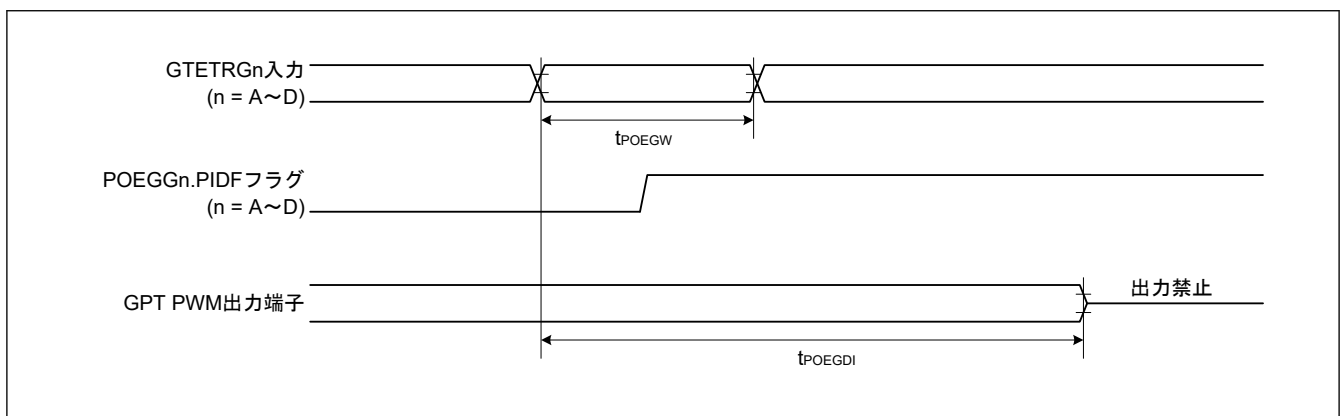
図 2.55 GTETRn 端子の入カレベル検出に対応した検出フラグによる POEG の出力禁止時間
