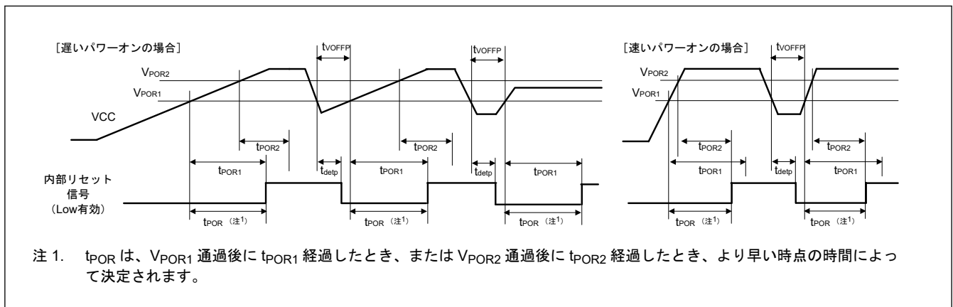
図 2.142 パワーオンリセットタイミング
