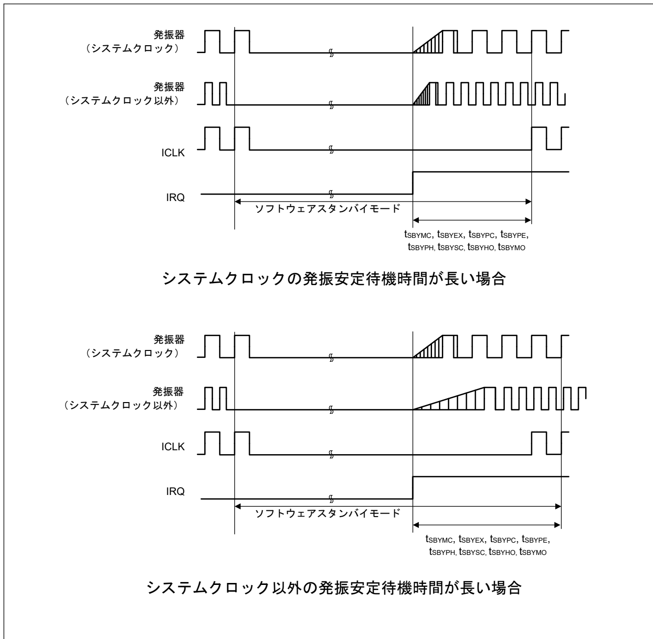
図 2.34 ソフトウェアスタンバイモード解除タイミング
