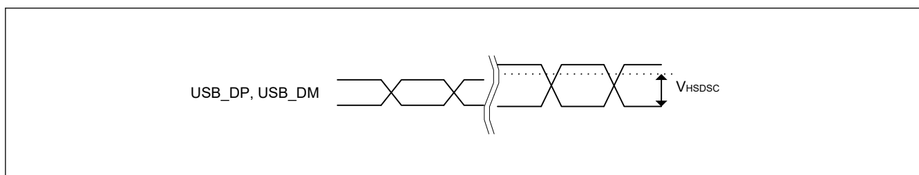
図 2.136 High-speed モードにおける USB_DP、USB_DM の切断検出感度
