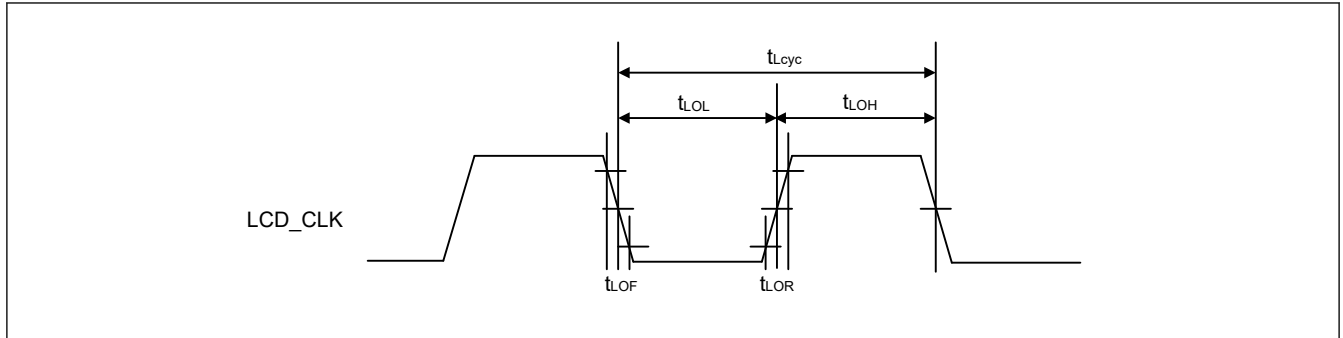
図 2.112 LCD_CLK クロック出力タイミング
