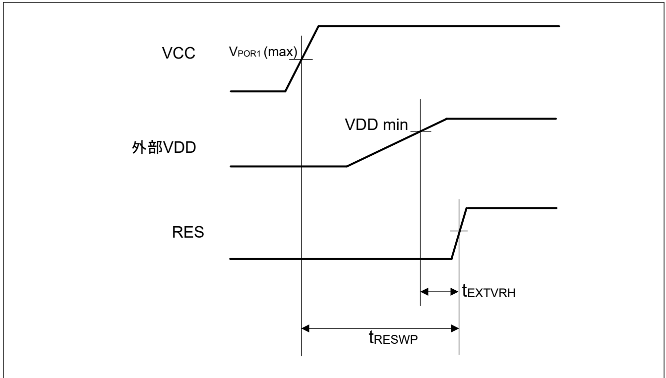
図 2.145 外部 VDD モードの電源起動シーケンス (RES 端子を使用する場合)
