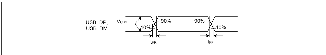
図 2.129 フルスピードモードにおける USB_DP、USB_DM の出カタイミング
