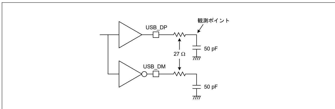
図 2.130 フルスピードモードにおける測定回路
