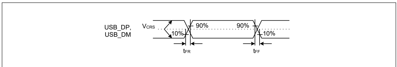
図 2.133 フルスピードモードにおける USB_DP、USB_DM の出カタイミング
