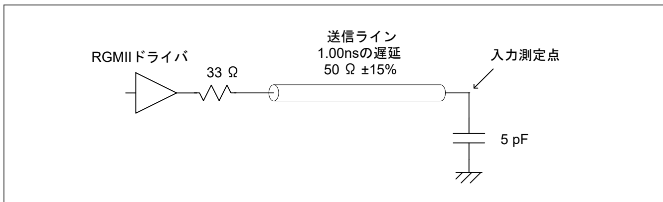
図 2.123 RGMII 出力タイミング計測条件
