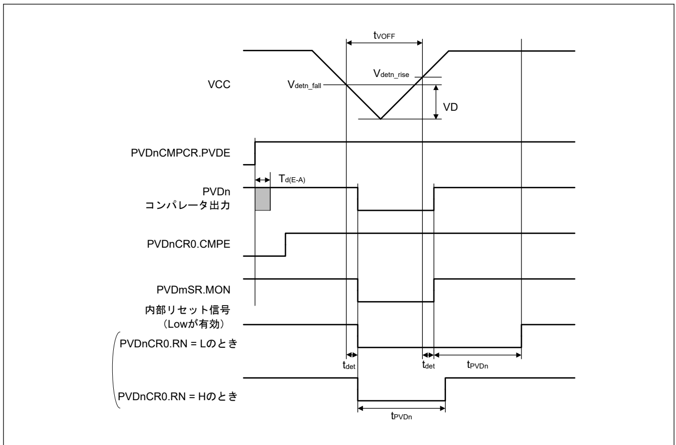
図 2.144 電圧検出回路タイミング ( V_{detn} ) ( n = 1, 2, 4, 5 )
