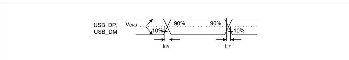
図 2.131 Low-speed モードにおける USB_DP、USB_DM の出力タイミング
