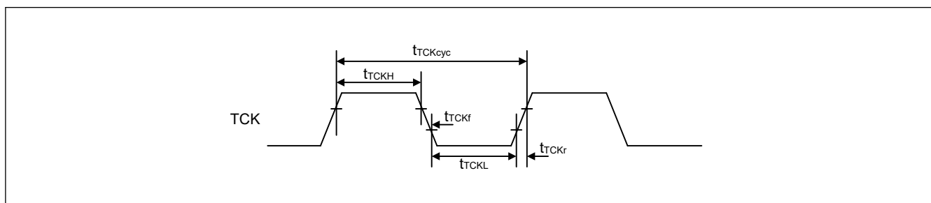
図 2.152 バウンダリスキャン TCK タイミング
