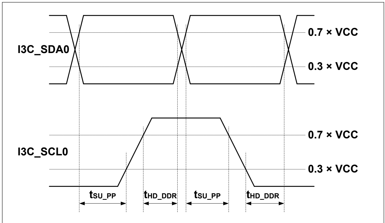
図 2.99 マスタ DDR タイミング
