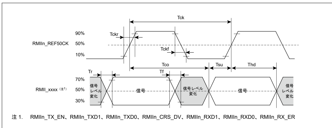
図 2.116 RMIIIn_REF50CK、RMII の信号タイミング
