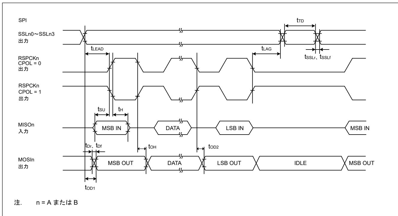
図 2.77 CPHA = 0 の場合におけるモトローラ SPI マスタの SPI タイミング
