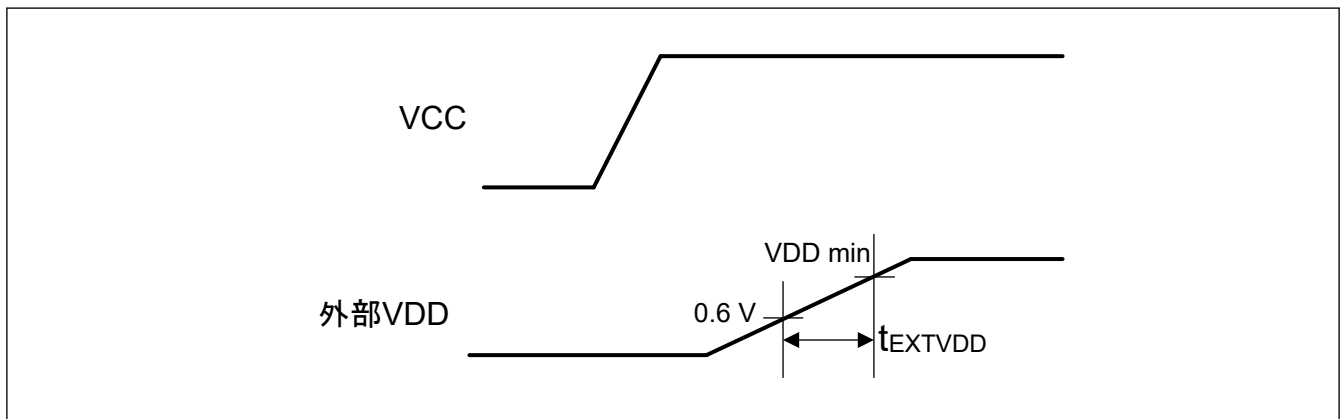
図 2.146 外部 VDD モードの電源起動シーケンス (RES 端子を使用しない場合)
