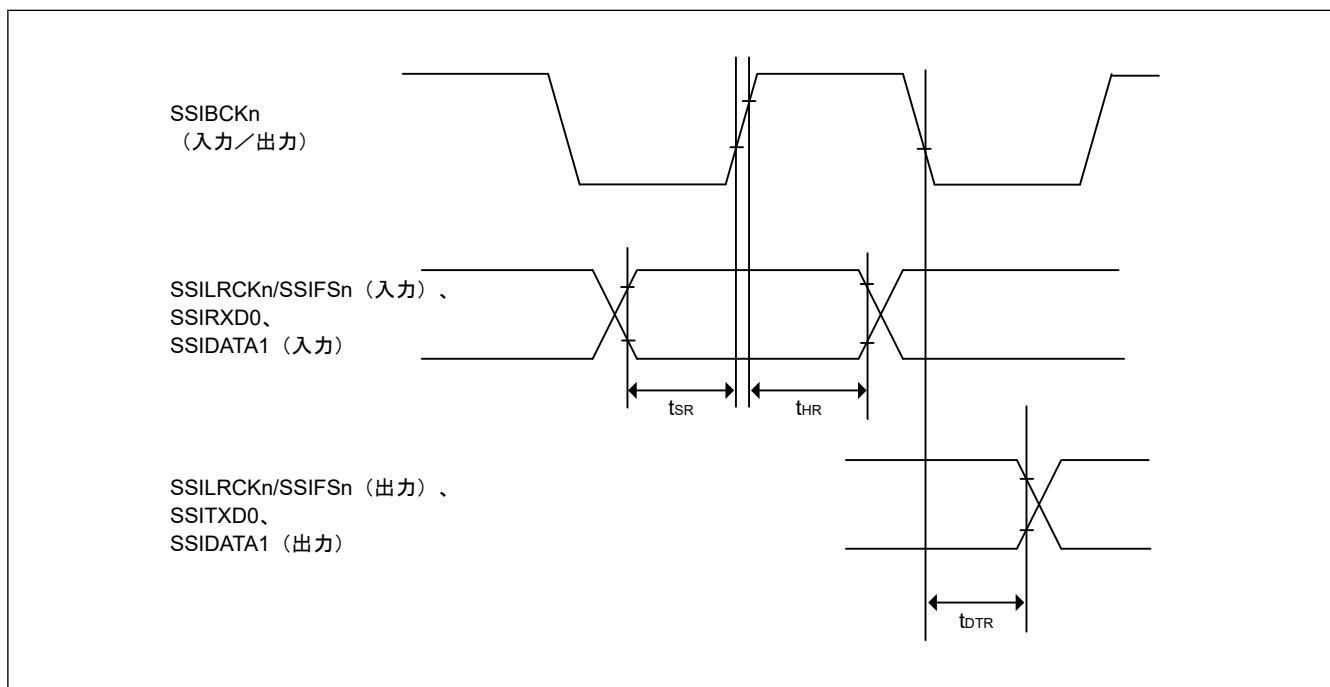
図 2.105 SSICR.BCKP = 0 の場合の SSIE データ送受信タイミング
