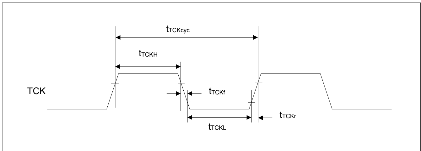
図 2.156 JTAG TCK タイミング
