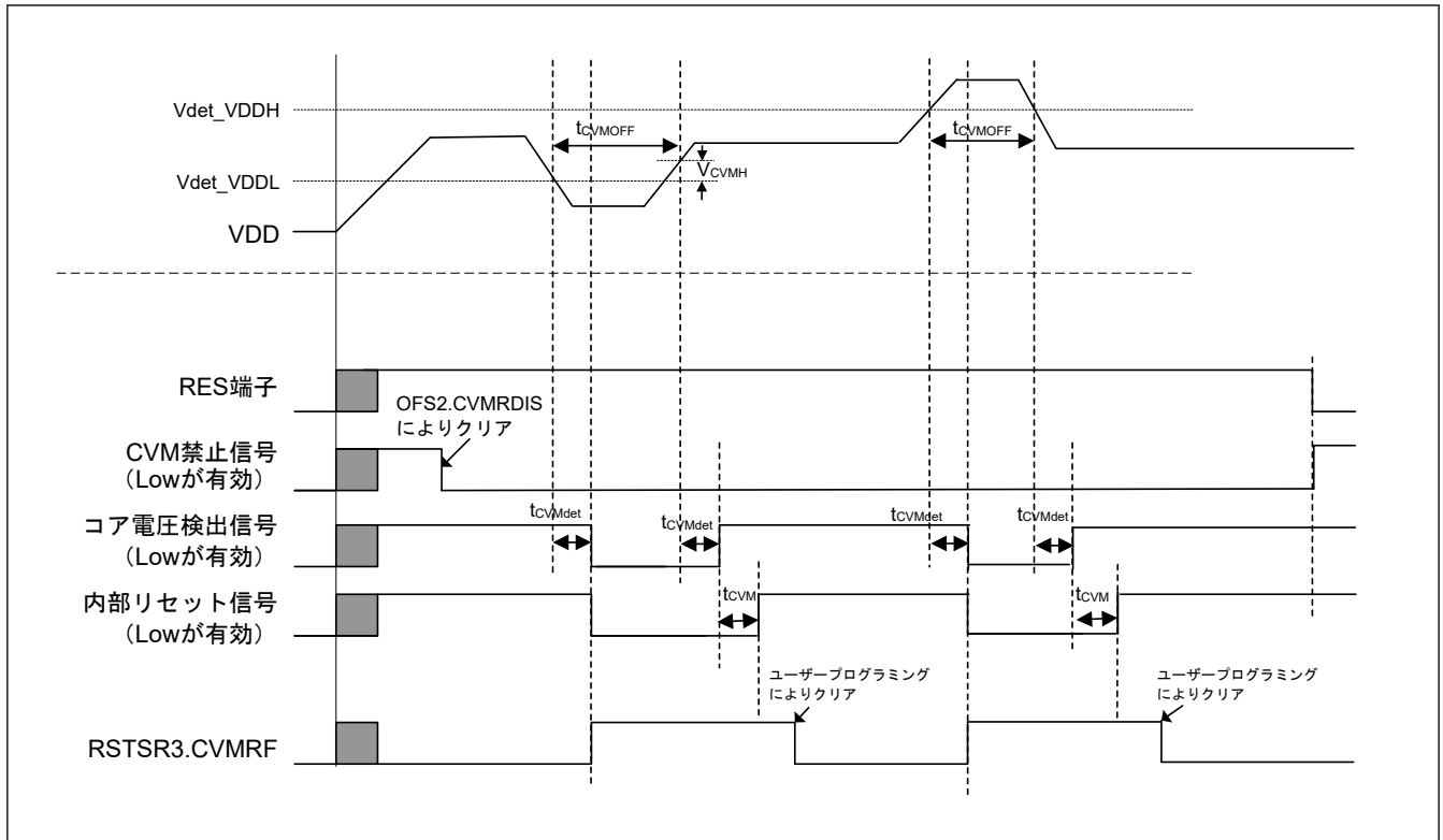
図 2.147 コア電圧監視リセット時間
