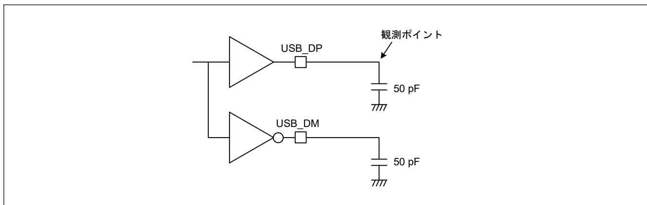
図 2.134 フルスピードモードにおける測定回路
