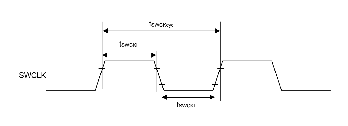
図 2.158 SWD SWCLK タイミング
