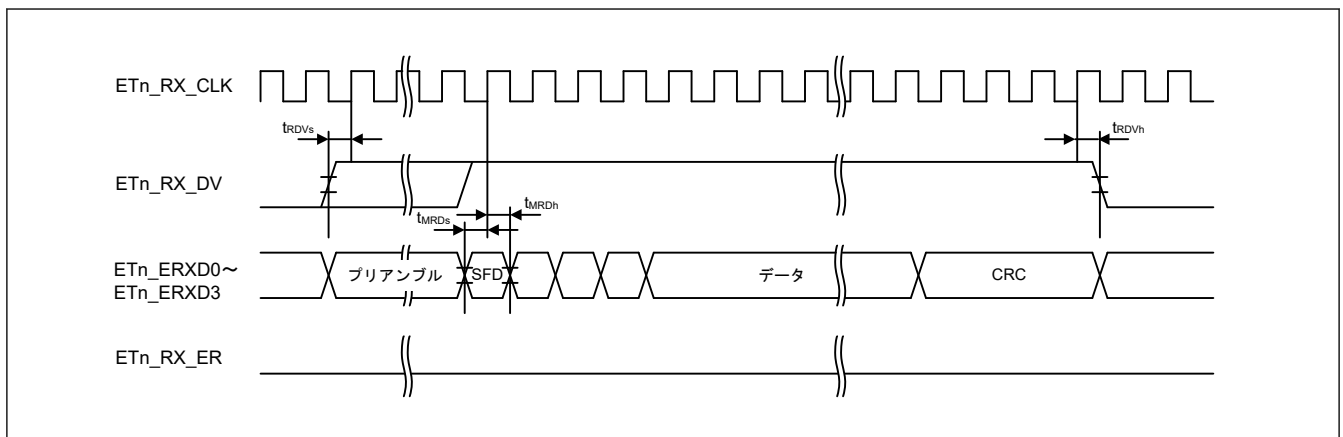
図 2.118 通常動作時の MII 受信タイミング
