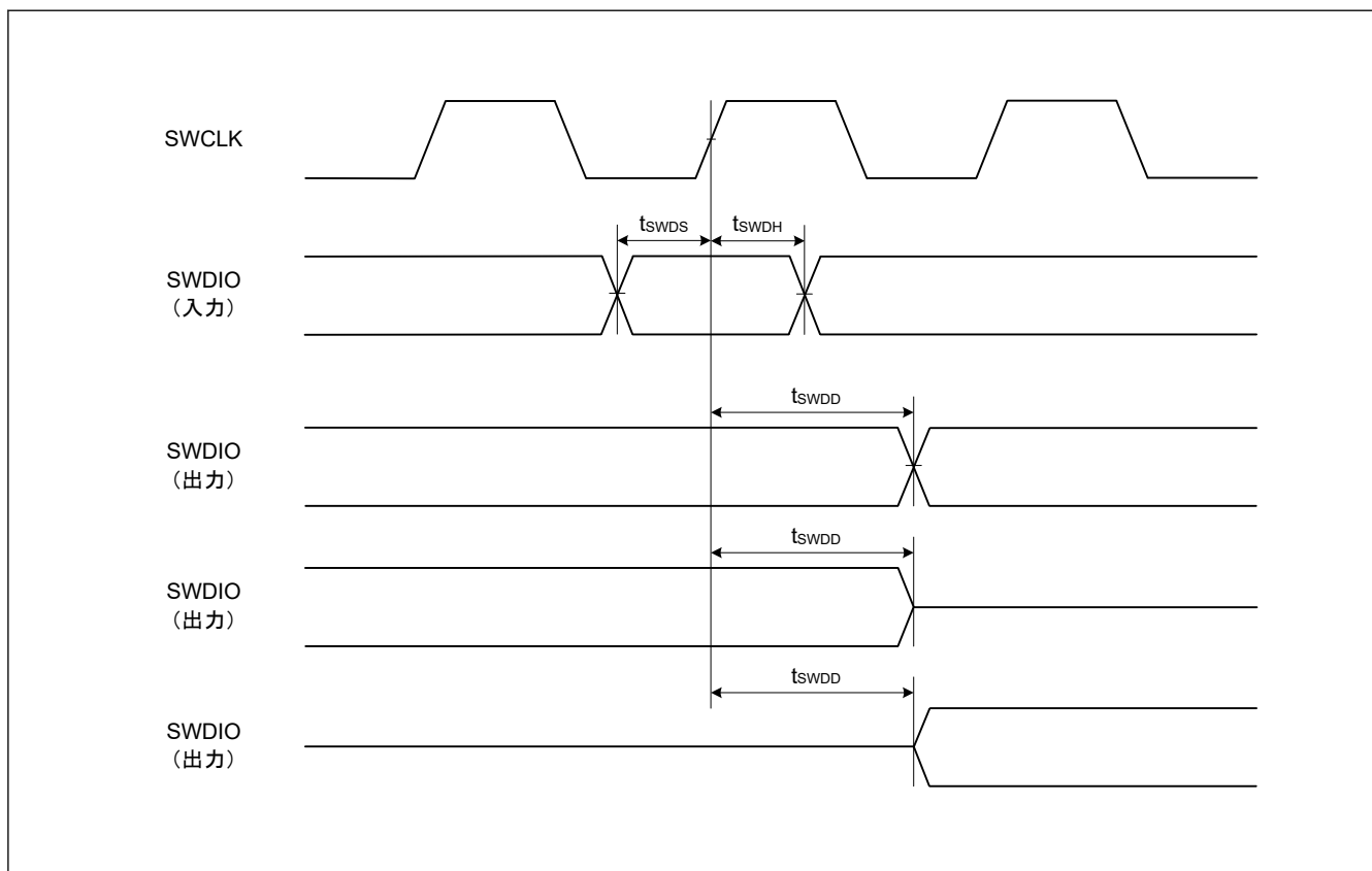
図 2.159 SWD 入出力タイミング
