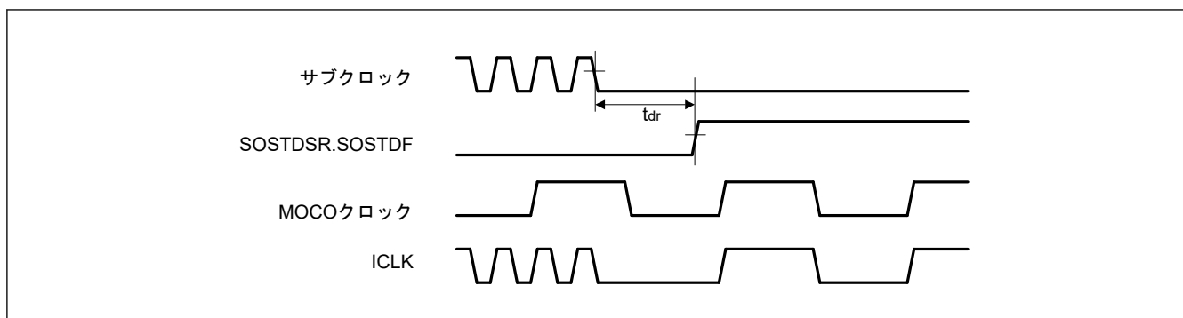
図 2.141 サブクロック発振器停止検出タイミング
