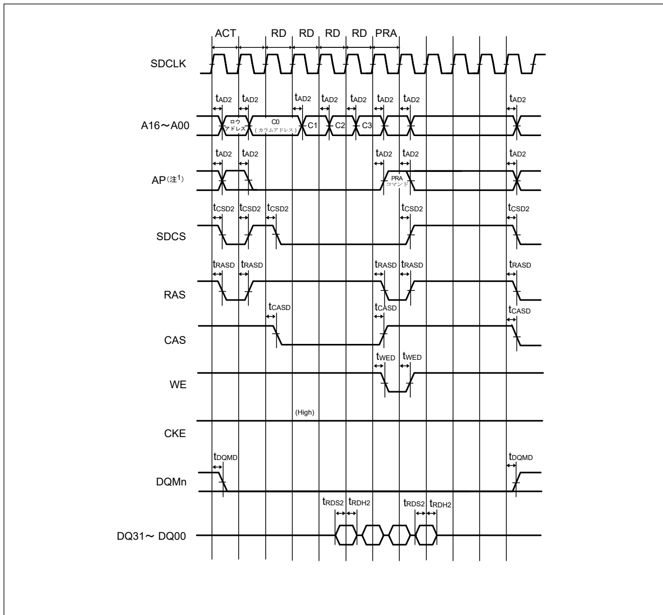
図 2.47 SDRAM マルチリードのタイミング
