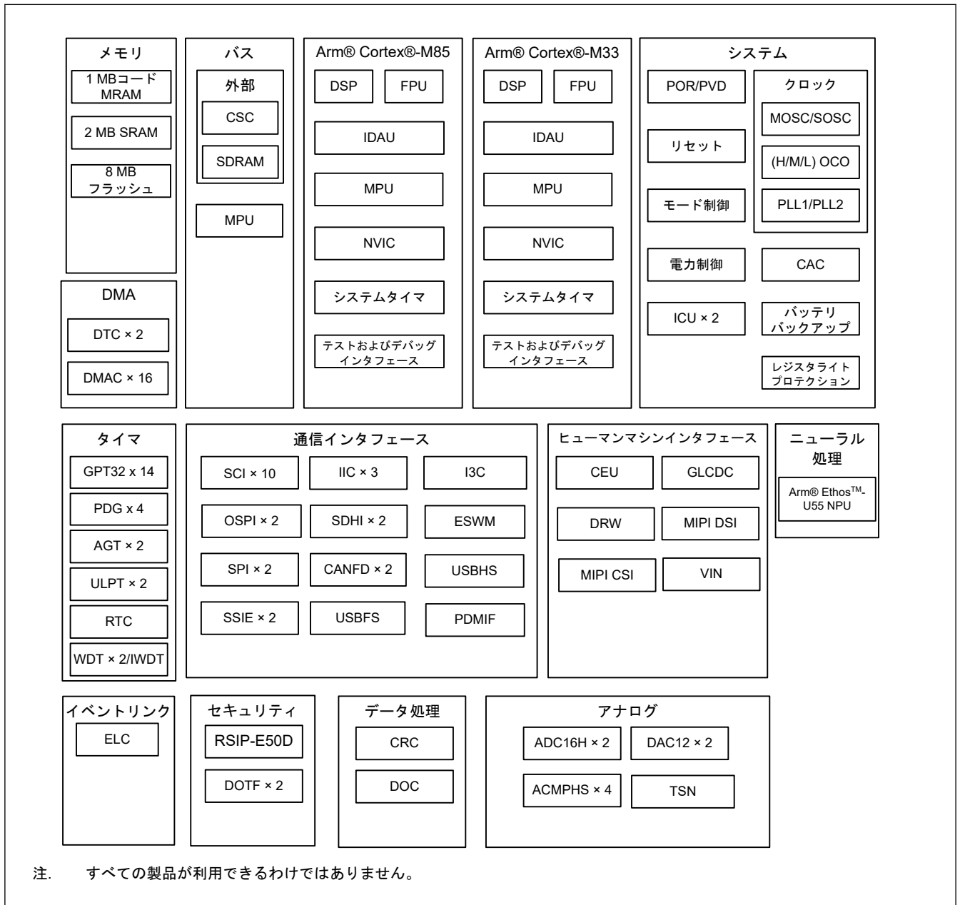
図 1.1 ブロック図
