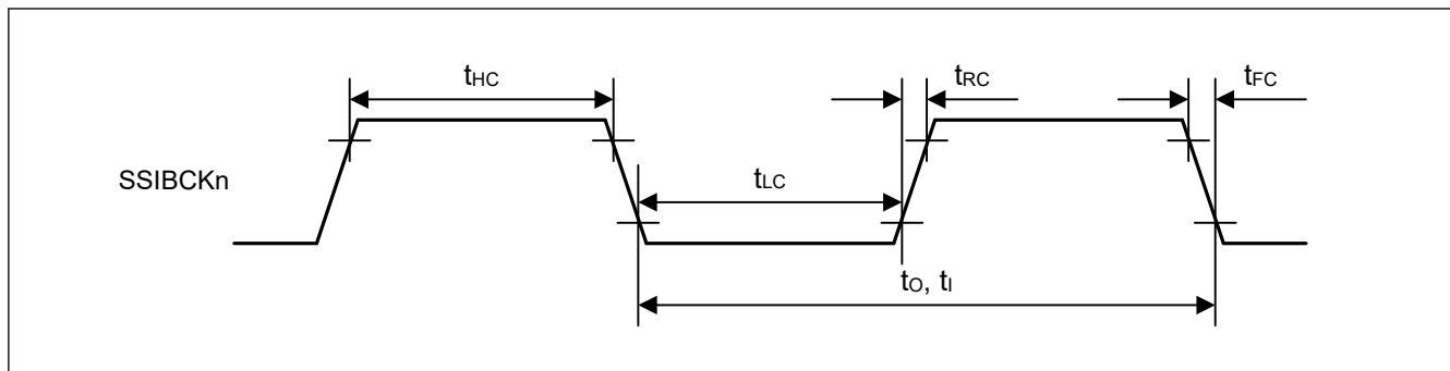
図 2.103 SSIE クロック入出力タイミング
