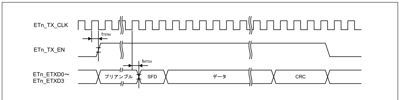
図 2.117 通常動作時の MII 送信タイミング
