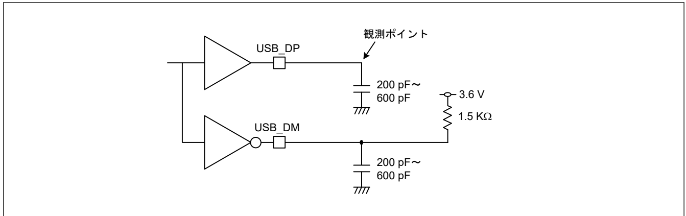
図 2.132 Low-speed モードにおける測定回路
