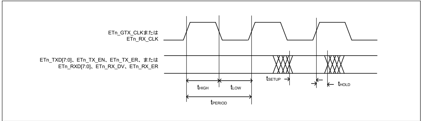
図 2.119 GMII タイミング
