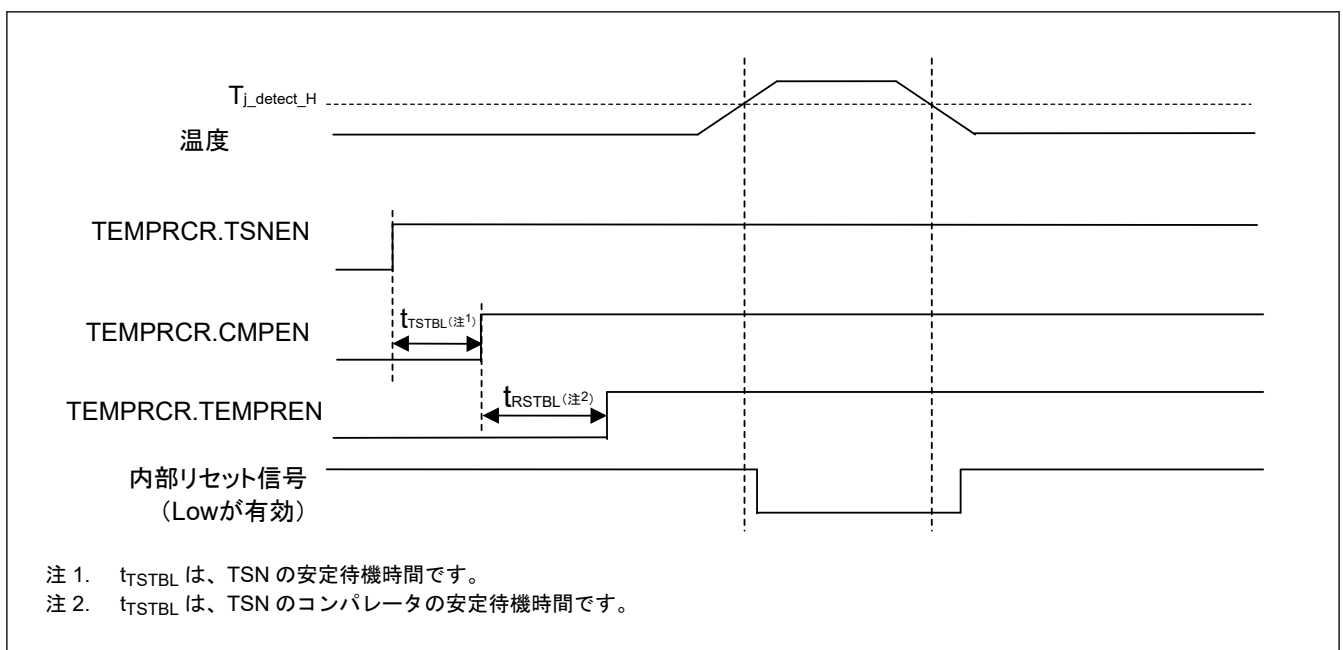
図 2.148 温度監視リセットのタイミング（高温検出）
