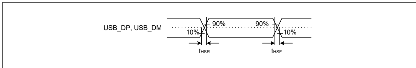
図 2.137 High-speed モードにおける USB_DP、USB_DM の出力タイミング
