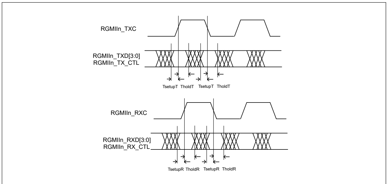
図 2.122 RGMII タイミング (RGMII-ID)
