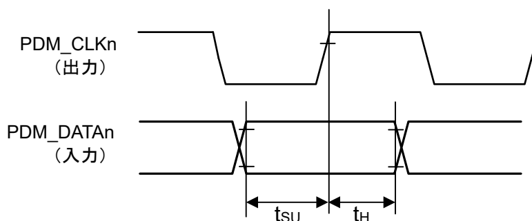
図 2.125 受信タイミング (PDM_CLKn の立ち上がりに同期)
