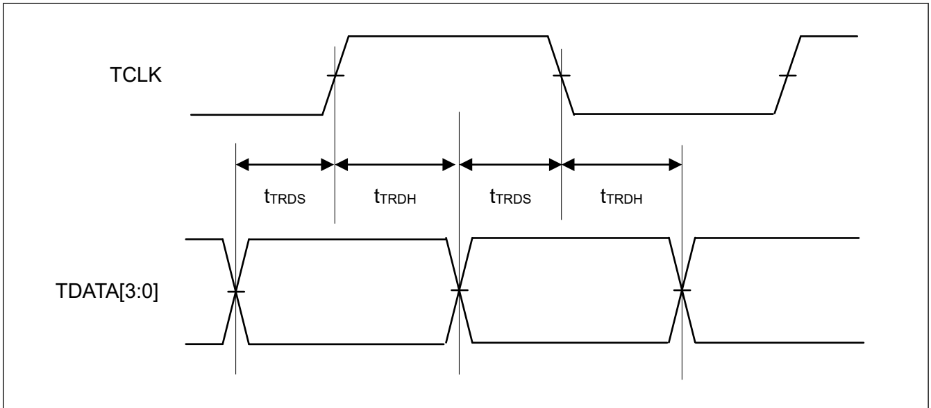
図 2.161 ETM 出力タイミング
