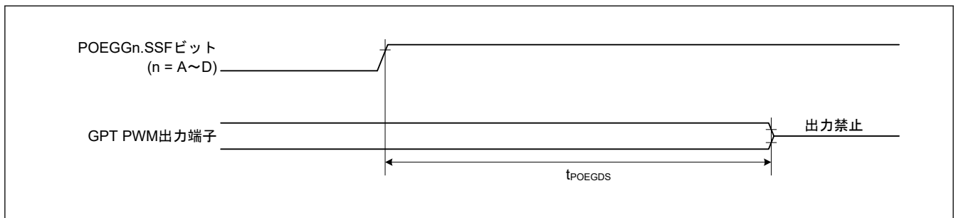
図 2.58 レジスタ設定に対応した POEG の出力禁止時間
