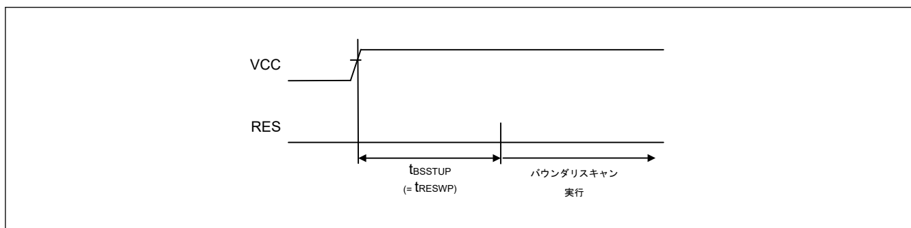
図 2.155 バウンダリスキャン回路起動タイミング
