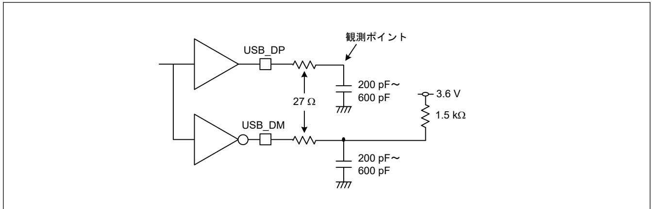
図 2.128 Low-speed モードにおける測定回路
