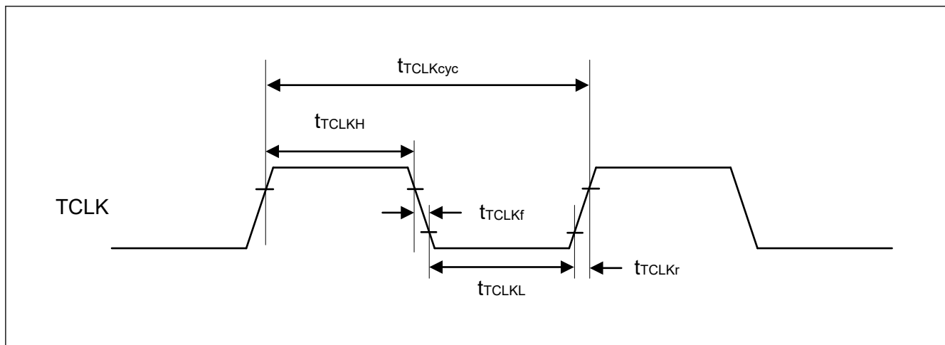
図 2.160 ETM TCLK タイミング
