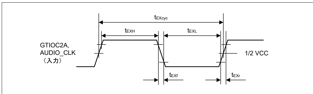
図 2.104 クロック入力タイミング
