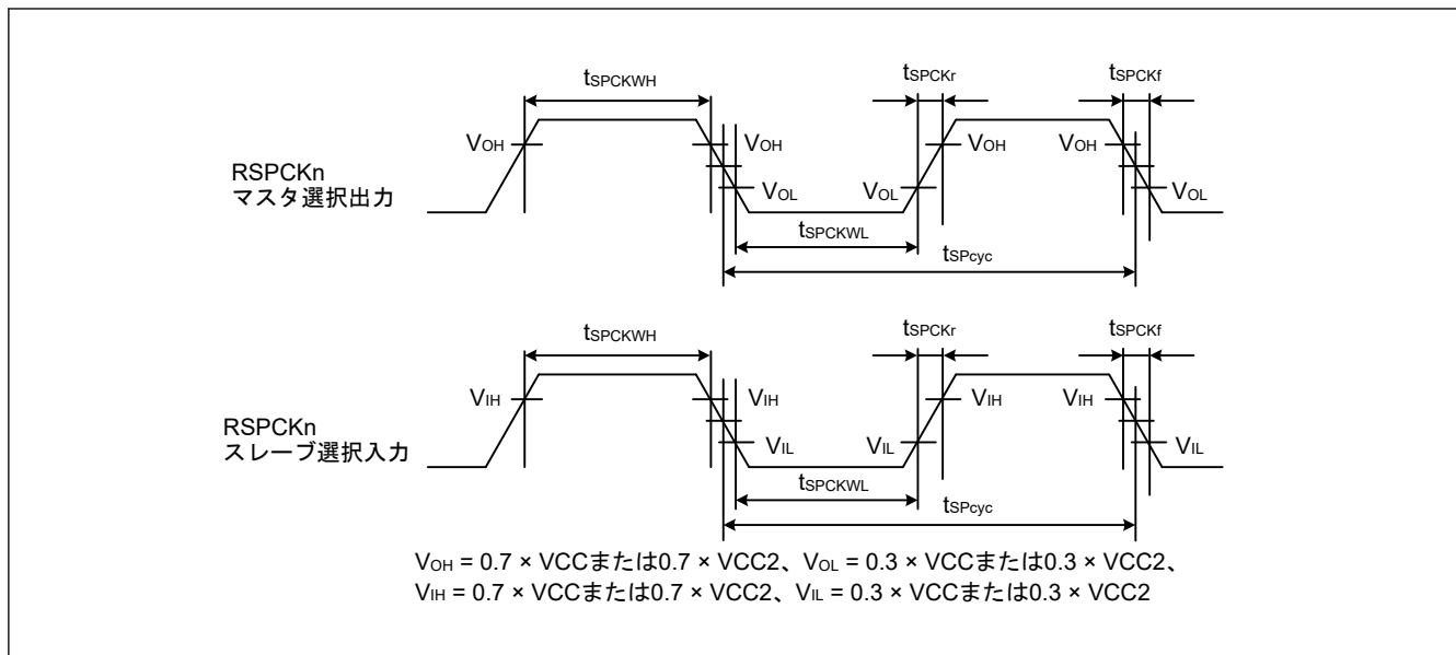
図 2.76 SPI クロックタイミング
