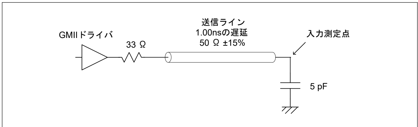
図 2.120 GMII 出力タイミング計測条件
