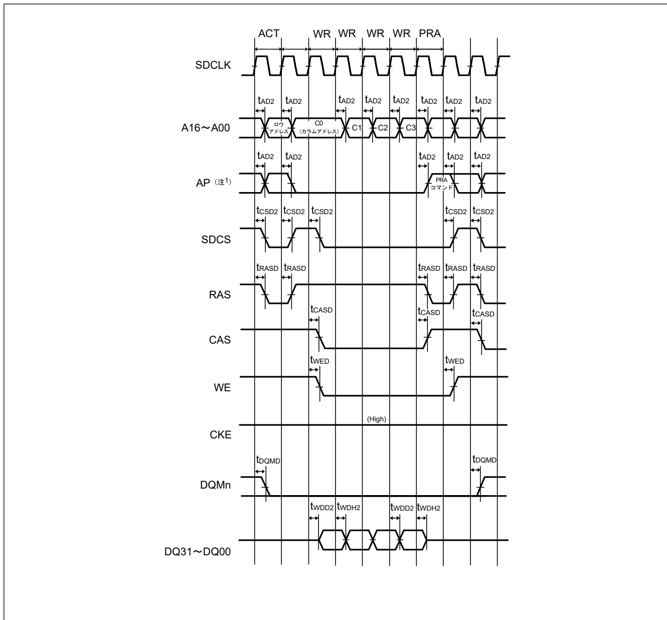
図 2.48 SDRAM マルチライトのタイミング
