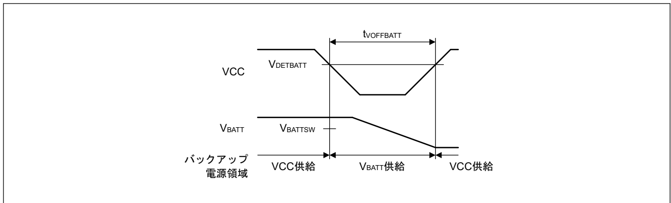
図 2.150 バッテリバックアップ機能特性
