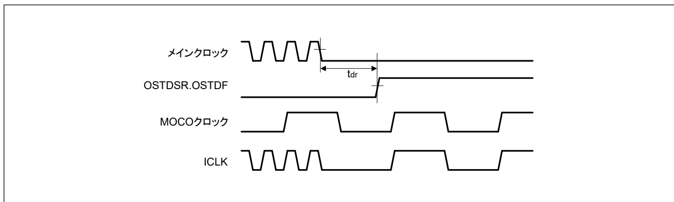
図 2.140 発振停止検出タイミング
