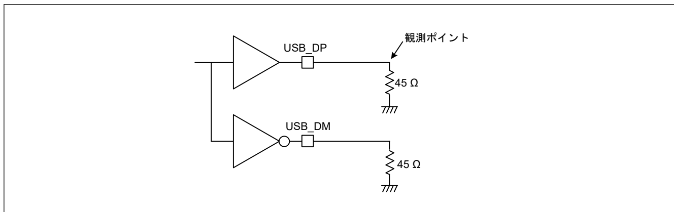
図 2.138 High-speed モードにおける測定回路
