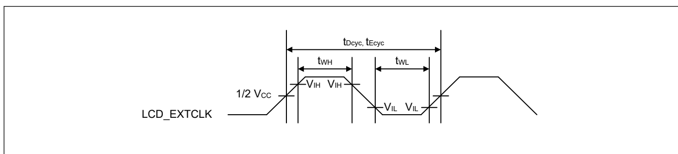
図 2.111 LCD_EXTCLK クロックタイミング
