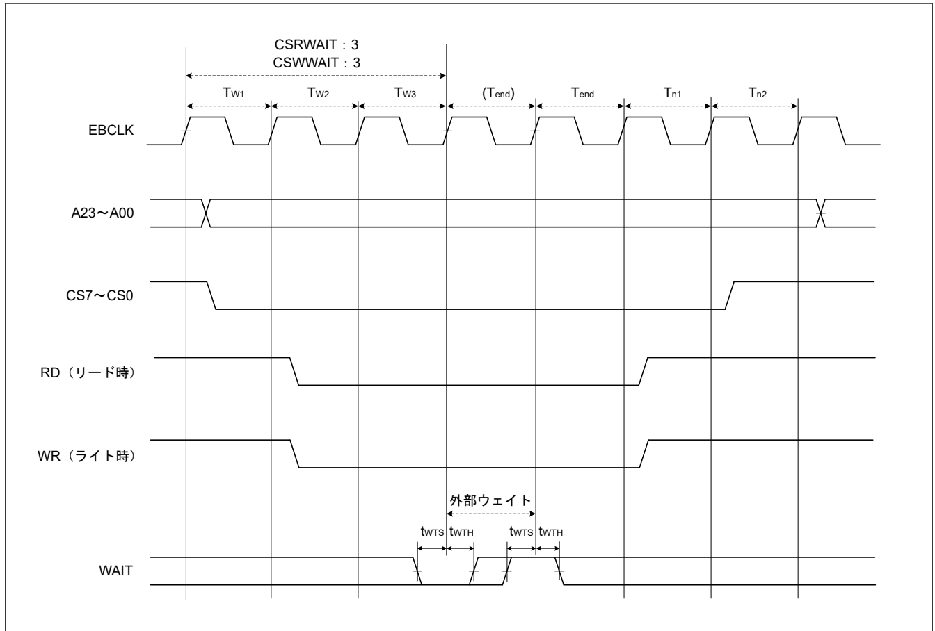
図 2.44 外部ウェイト制御の外部パスタイミング
