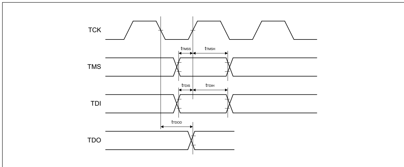
図 2.153 バウンダリスキャン入出力タイミング (1)
