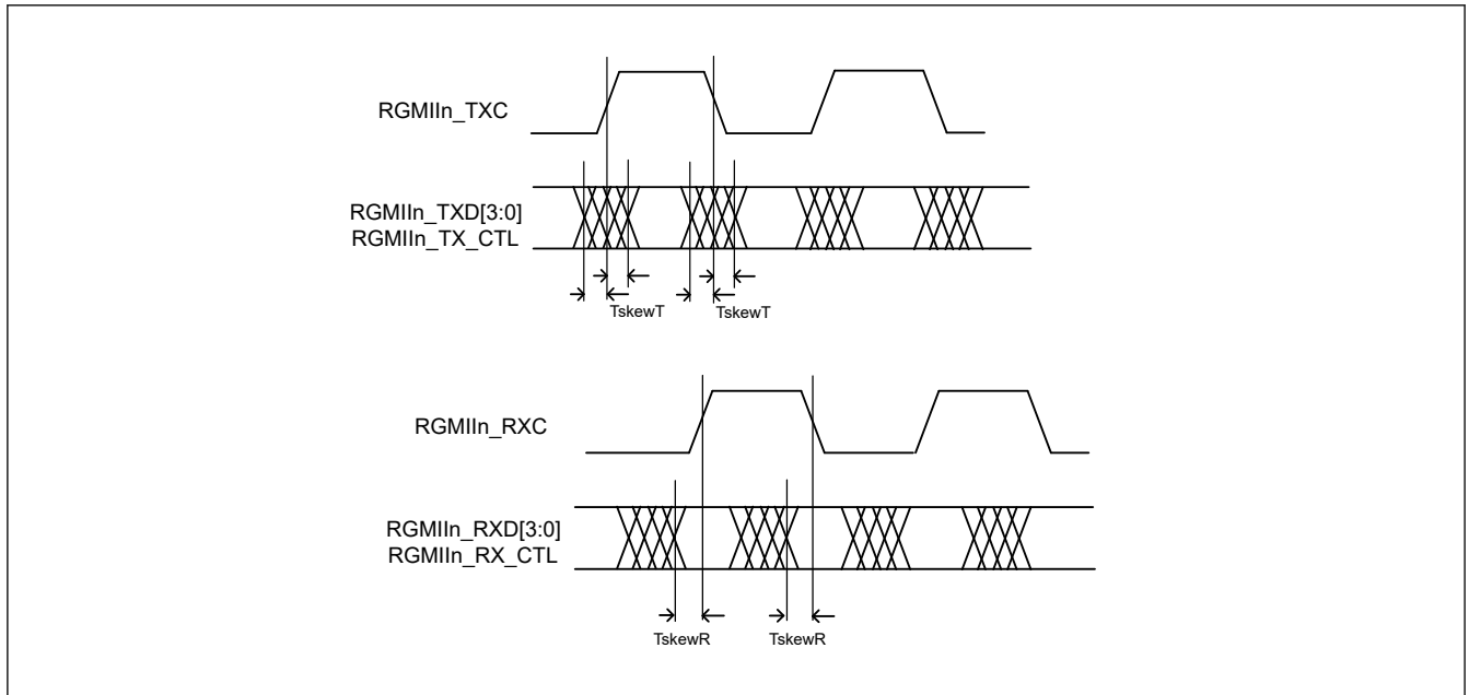
図 2.121 RGMII タイミング
