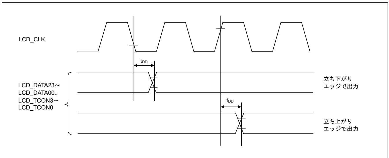
図 2.113 表示出力タイミング
