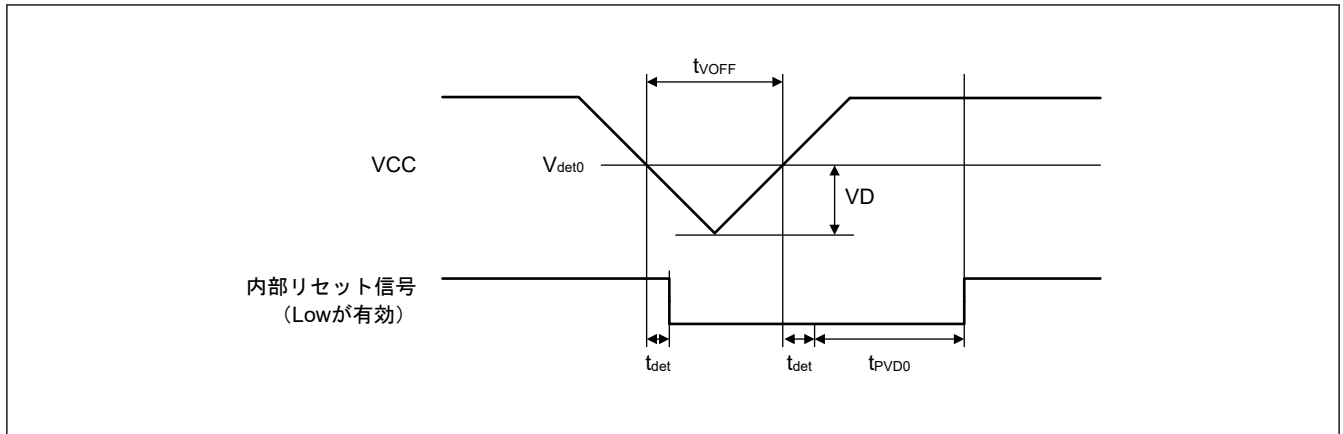
図 2.143 電圧検出回路タイミング ( V_{det0} )
