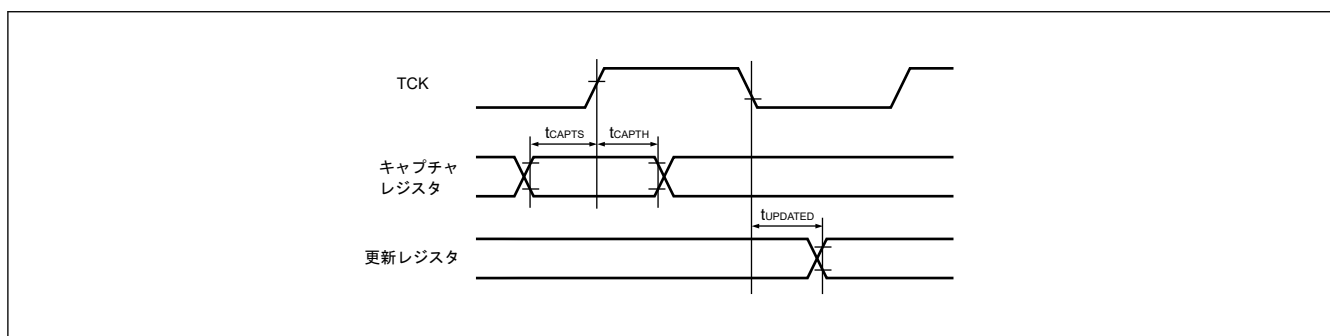
図 2.154 バウンダリスキャン入出力タイミング (2)
