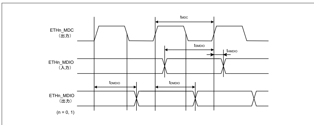
図 2.124 ETn_MDIO、ETn_MDC タイミング
