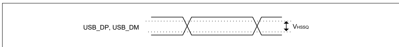
図 2.135 High-speed モードにおける USB_DP、USB_DM の Squelch 検出感度
