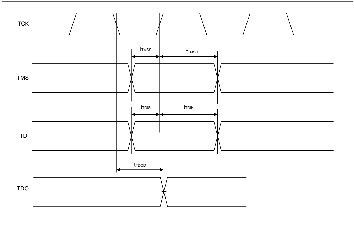
図 2.157 JTAG 入出力タイミング
