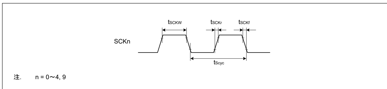
図 2.69 SCK クロック入出力タイミング
