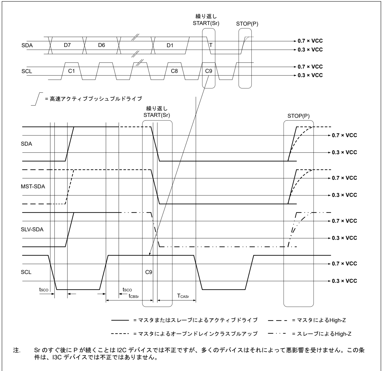
図 2.100 繰り返しのスタートコンディションおよびストップコンディションでのマスタ終了時の T ビット読み出し
