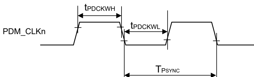
図 2.124 クロック出力のタイミング (PDM_CLKn)
