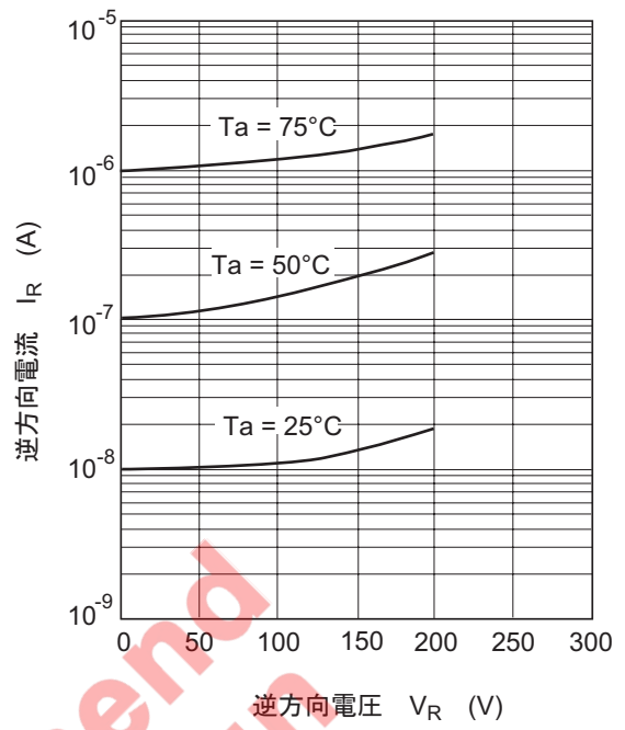
图2. 逆方向特性
