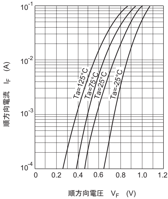
图1. 顺方向特性
