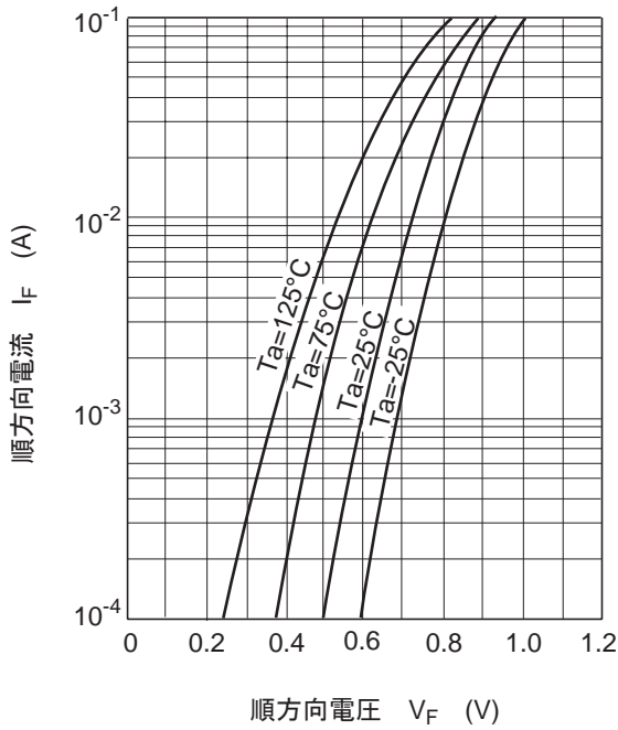
图1. 顺方向特性
