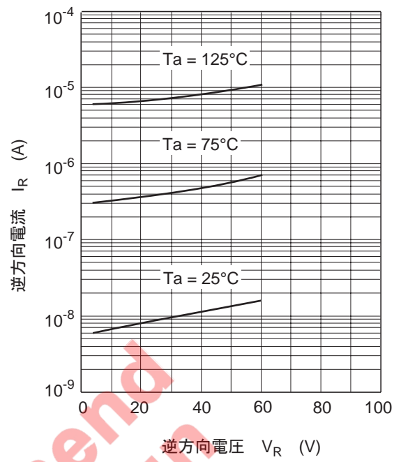
图2. 逆方向特性
