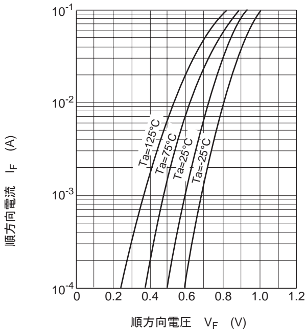
图1. 顺方向特性
