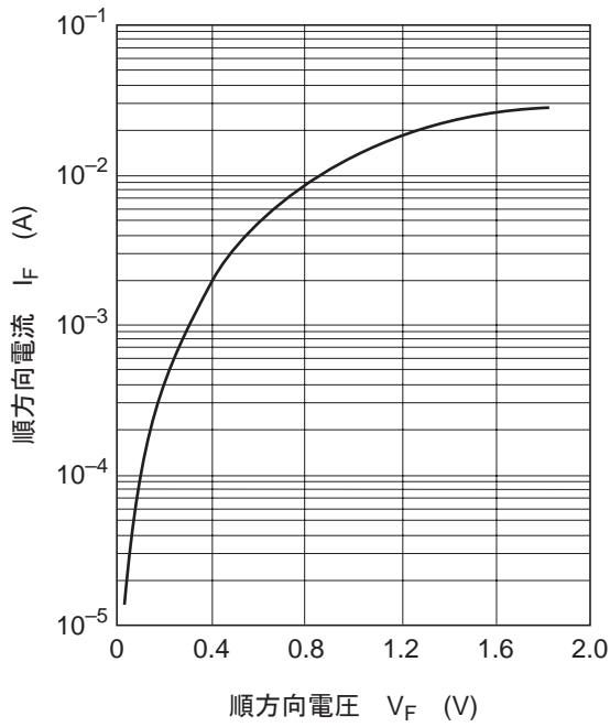
图1. 順方向特性
