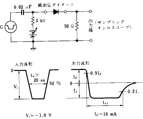
t_{rr} 測定回路と波形定義
