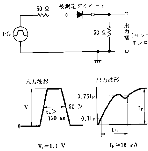
t_{fr} 測定回路と波形定義
