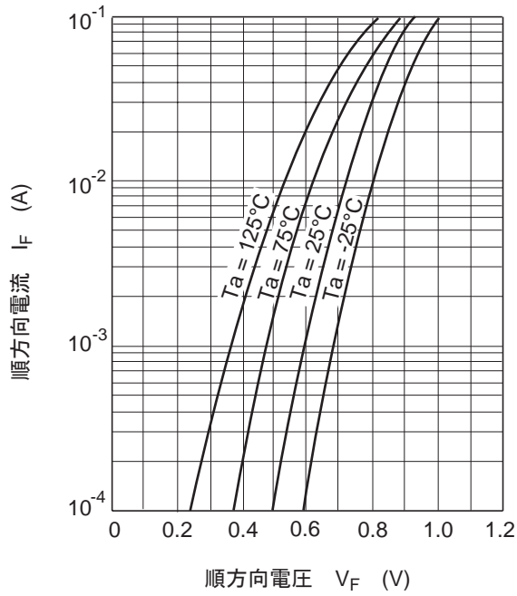
図1. 順方向特性
