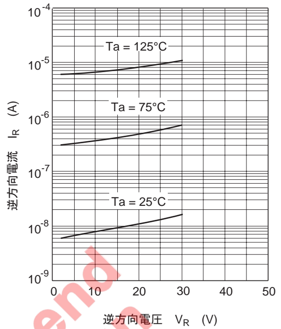
図2. 逆方向特性
