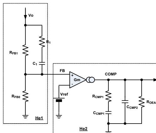
図 52. タイプ III 補償回路
