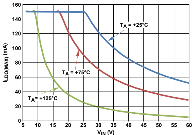
図 47. 電力ディレーティング曲線
