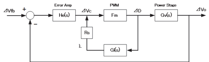
図 50. 概念制御ブロック図
