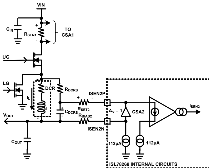
図 45. インダクタ DCR 電流センス
