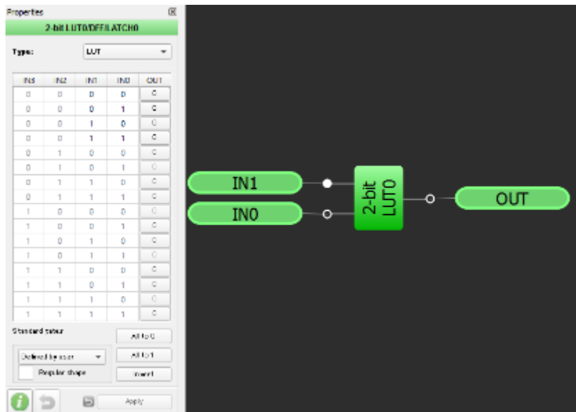
コンビネーション・ファンクション・マクロセル 2-bit LUT を選択した場合
