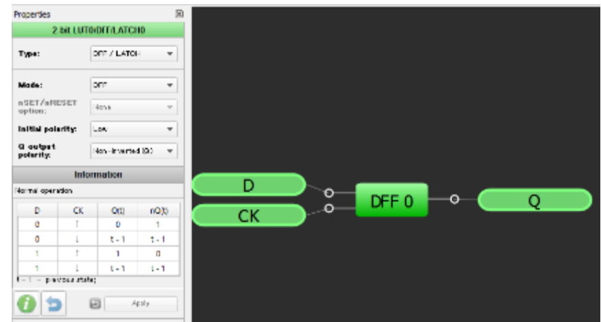
コンビネーション・ファンクション・マクロセル DFF を選択した場合
